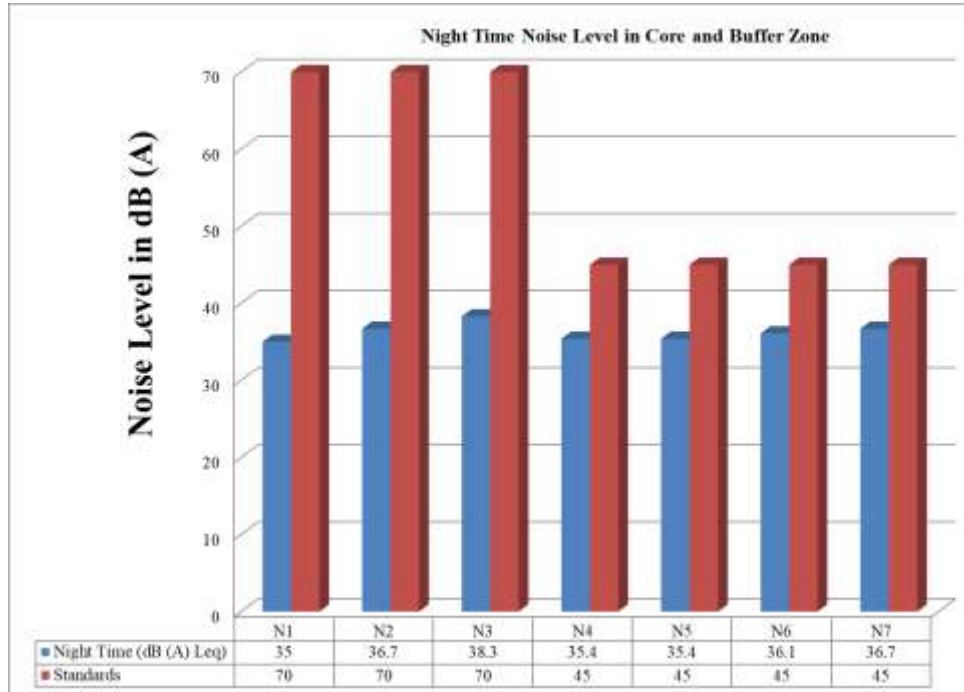
படம் 3.26: முக்கிய மற்றும் இடையக மண்டலத்தில் இரவு நேர இரைச்சல் நிலைகள்
