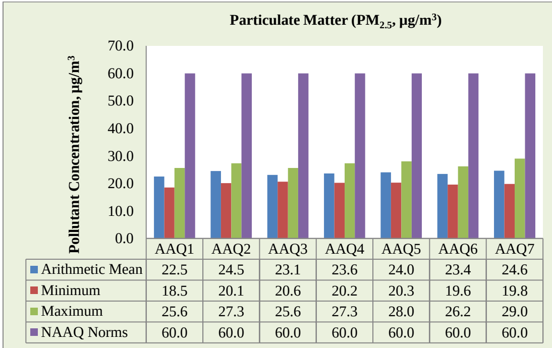
படம் 3.18: பார்டிகுலேட் மேட்டரின் பார் வரைபடம் PM 2.5
