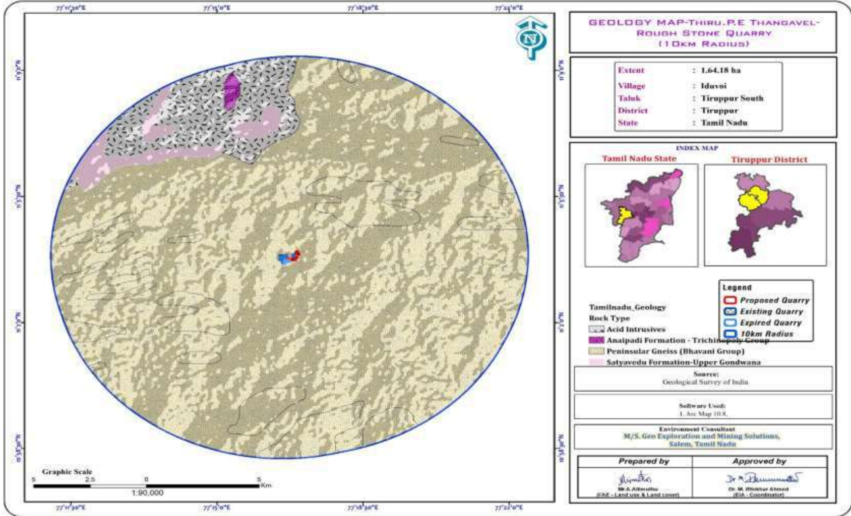
படம் 2.7 மண்டல புனியியல் வரைபடம்
