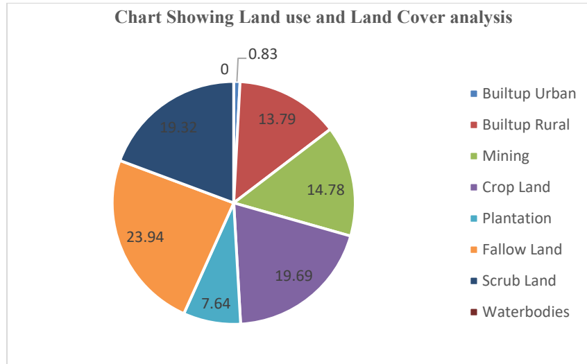
படம் 3.1: LISS III தரவைப் பயன்படுத்தி நிலப்பரப்பு/நிலப்பரப்பு பகுப்பாய்வு
