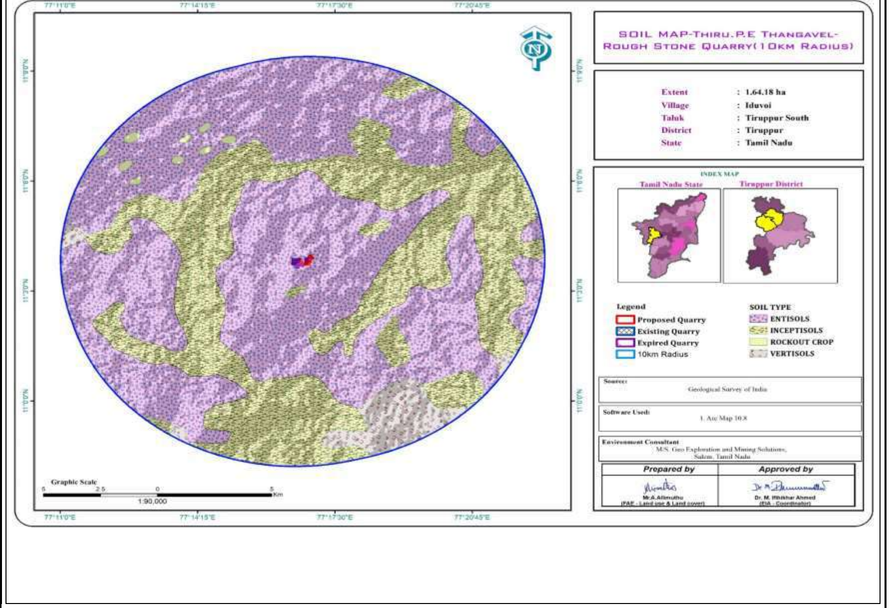
படம் 3.6: மண் வரைபடம்
