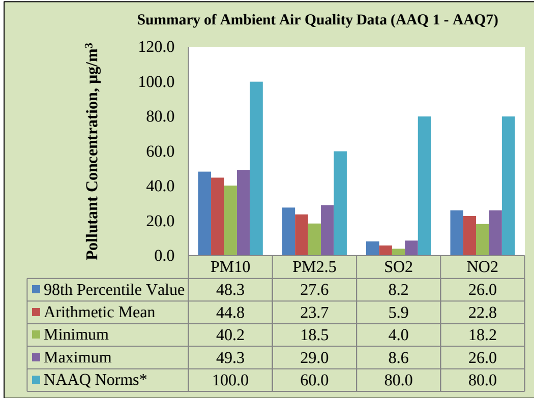
படம் 3.17: AAQ1 - AAQ7 இன் சுருக்கத்தின் பட்டி வரைபடம்
