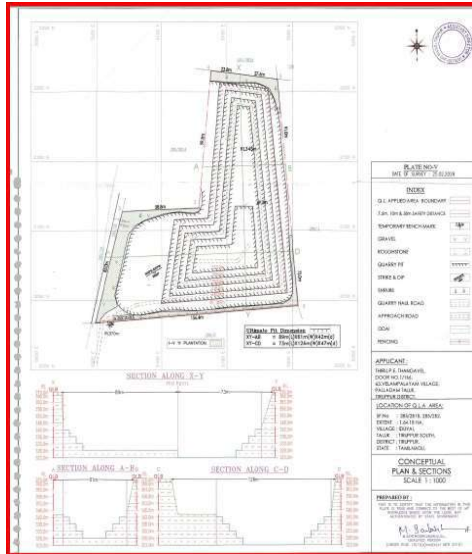
படம் 2.11: சுரங்க மூடல் திட்டம் மற்றும் பிரிவுகள்
