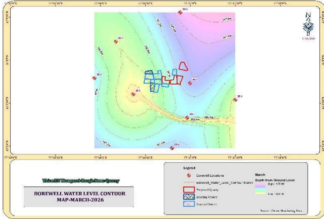
படம் 3.11: ஆழ்துளைக் கிணறுகளின் வரைபடம் - மார்ச் முதல் மே 2026 வரை
