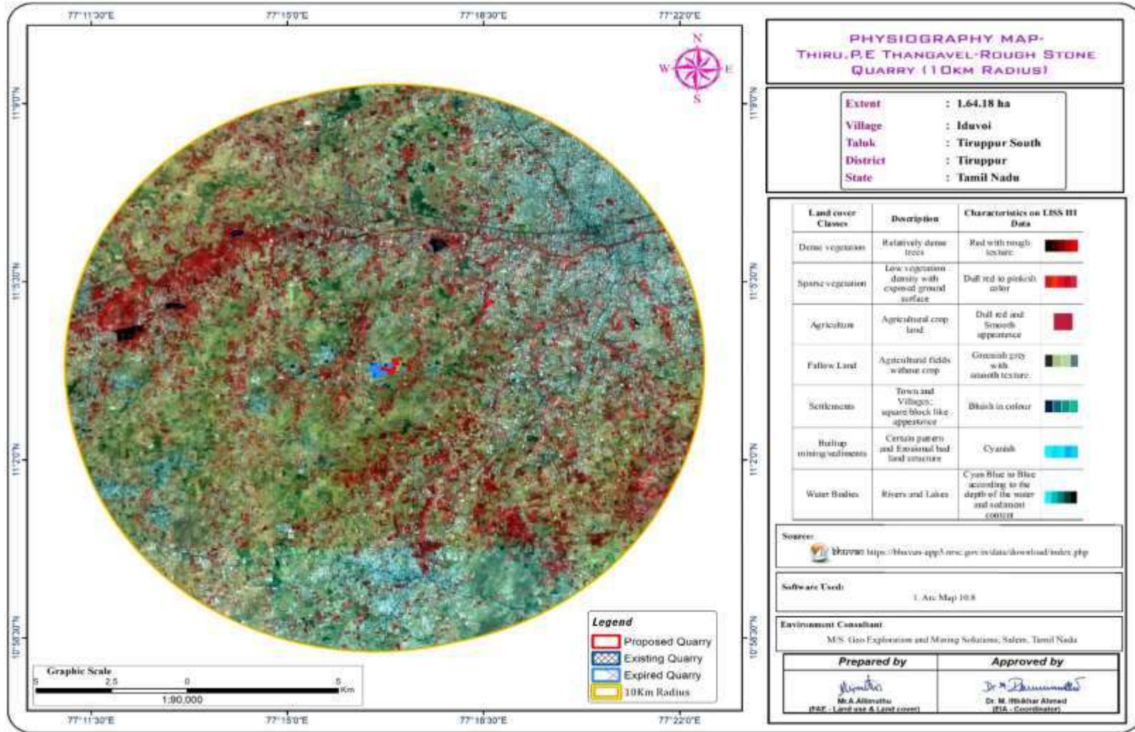
படம் 3.2: பிசியோகிராஃபிக் வரைபடம் 10 கிமீ சுற்றளவு
