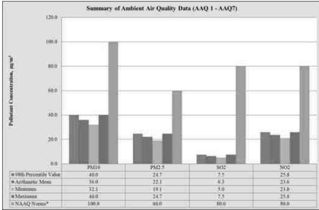
படம் 3.17: AAQ1 – AAQ7 இன் சுருக்கத்தின் பட்டி வரைபடம்
