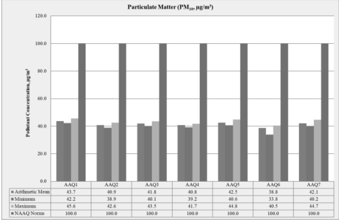
படம் 3.16: பார்டிகுலேட் மேட்டரின் பார் வரைபடம் PM 10
