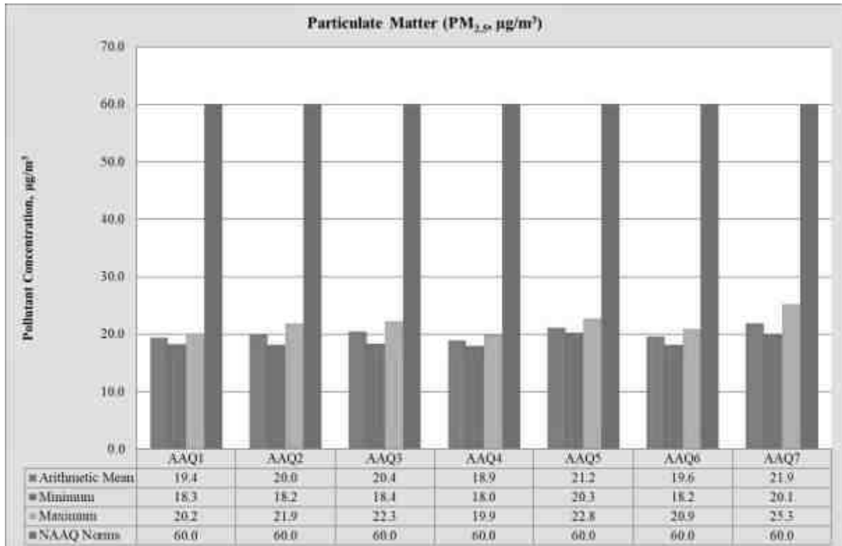
படம் 3.15: பார்டிகுலேட் மேட்டரின் பார் வரைபடம் PM 2.5
