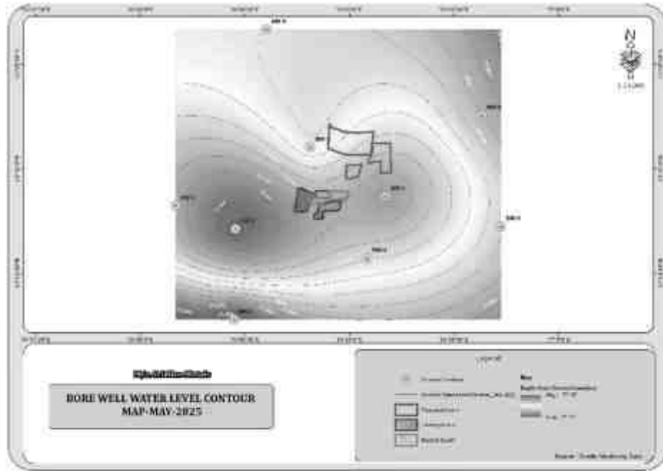
படம் 3.11: ஆழ்துளைக் கிணறுகளின் வரைபடம் - மே 2025
