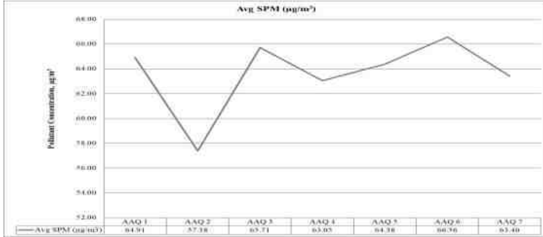
படம் 3.19: சராசரி SPM மதிப்புகளின் வரி வரைபடம்
