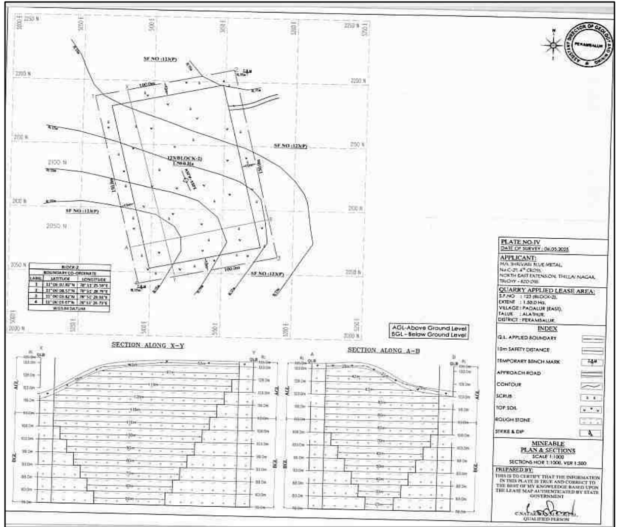
படம் 2.7 சுரங்கத் திட்டம் & பிரிவுகள்
