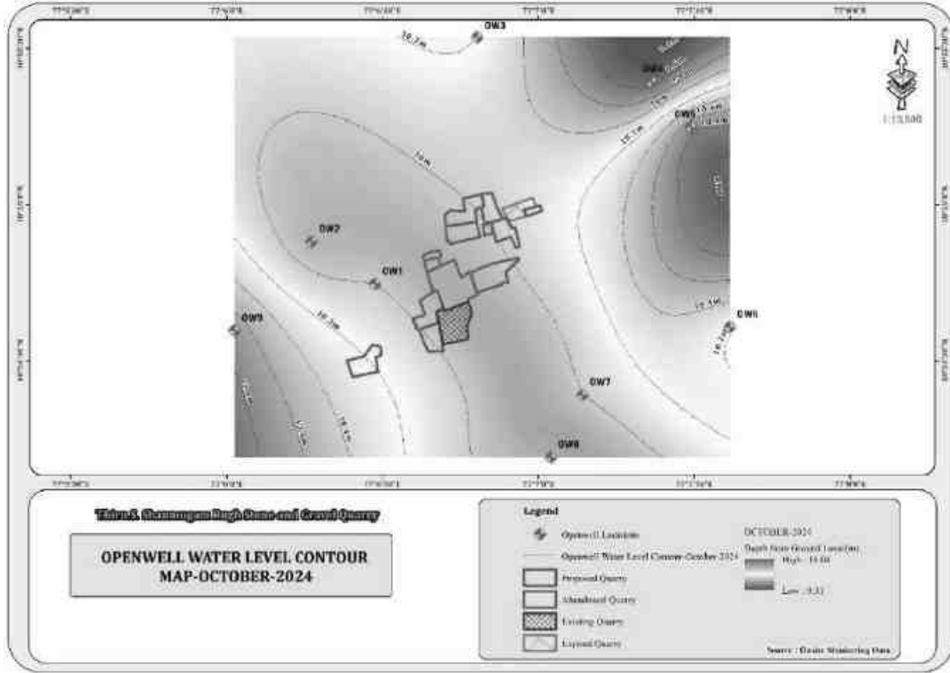
படம் 3.6: திறந்தவெளி கிணற்று நீர் மட்டத்தின் விளிம்பு வரைபடம்
