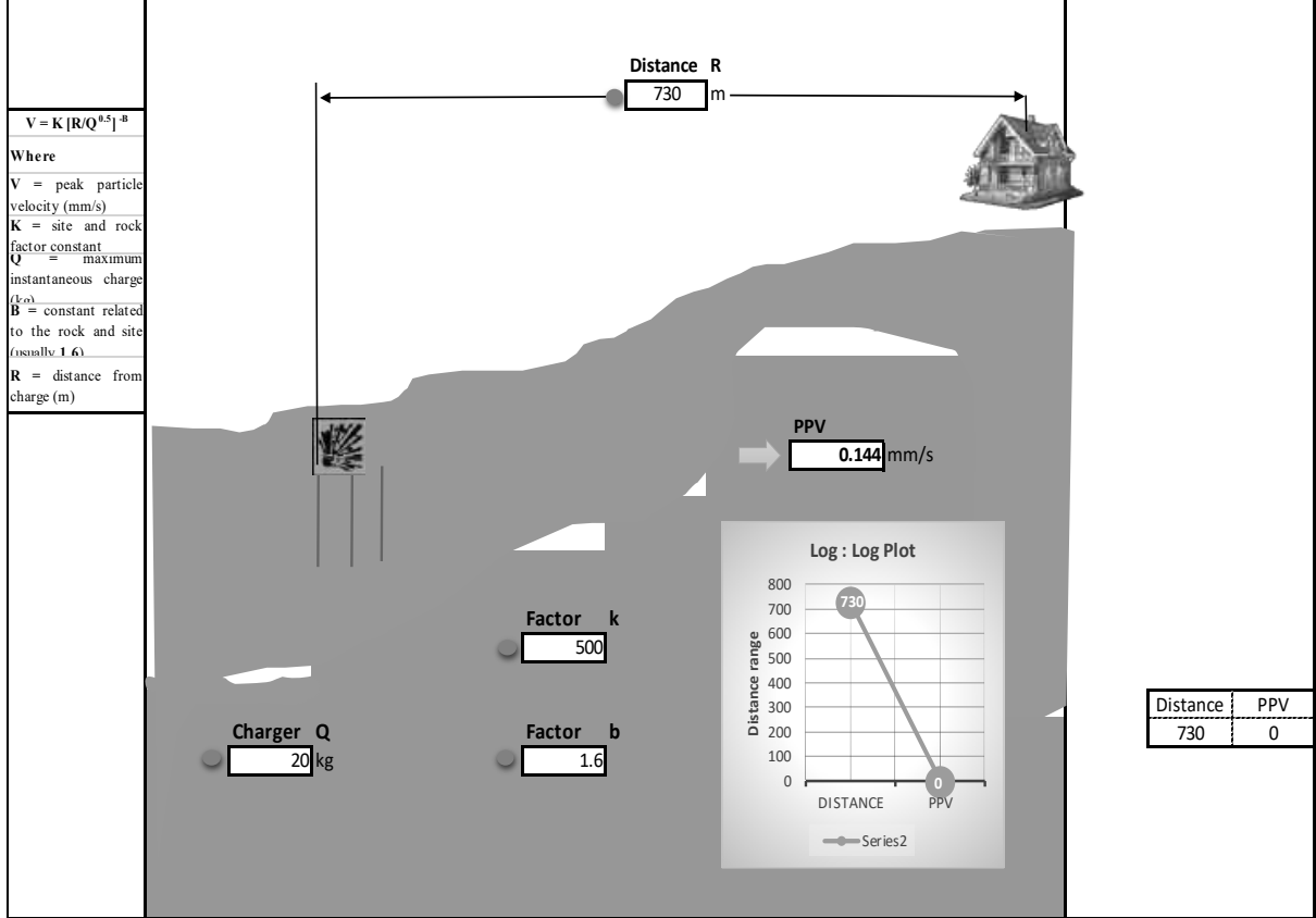
படம் 4.6: நில அதிர்வு கணிப்பு
