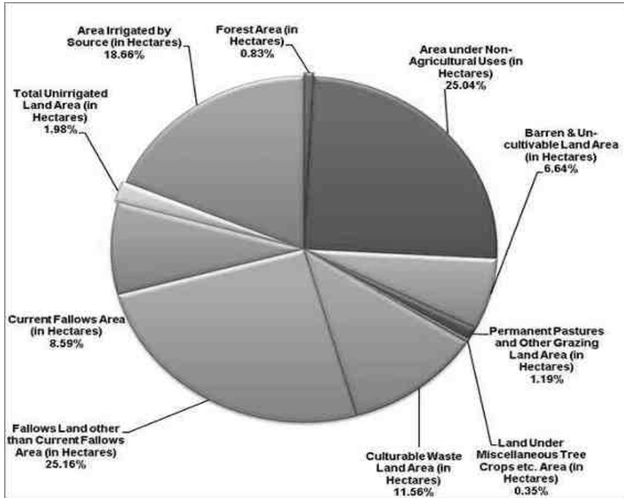
படம் 3.10.A- நில பயன்பாட்டு முறை இடையக மண்டலத்திற்குள்
