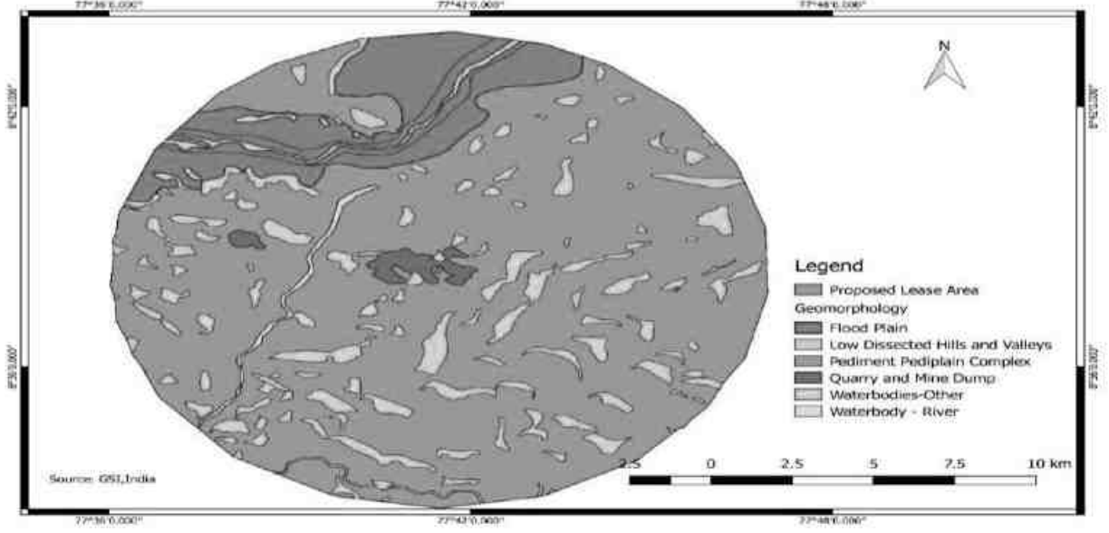
படம் 3.14 ஆய்வுப் பகுதியின் புவிபியல்
