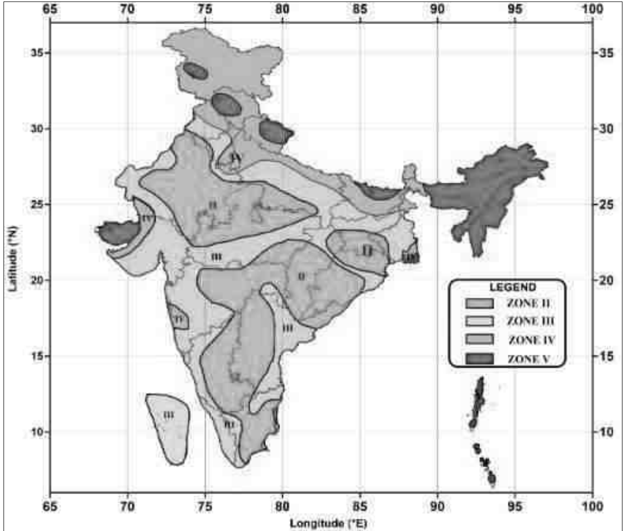
படம் 3.3 - இந்தியாவின் நில அதிர்வு வரைபடம்
