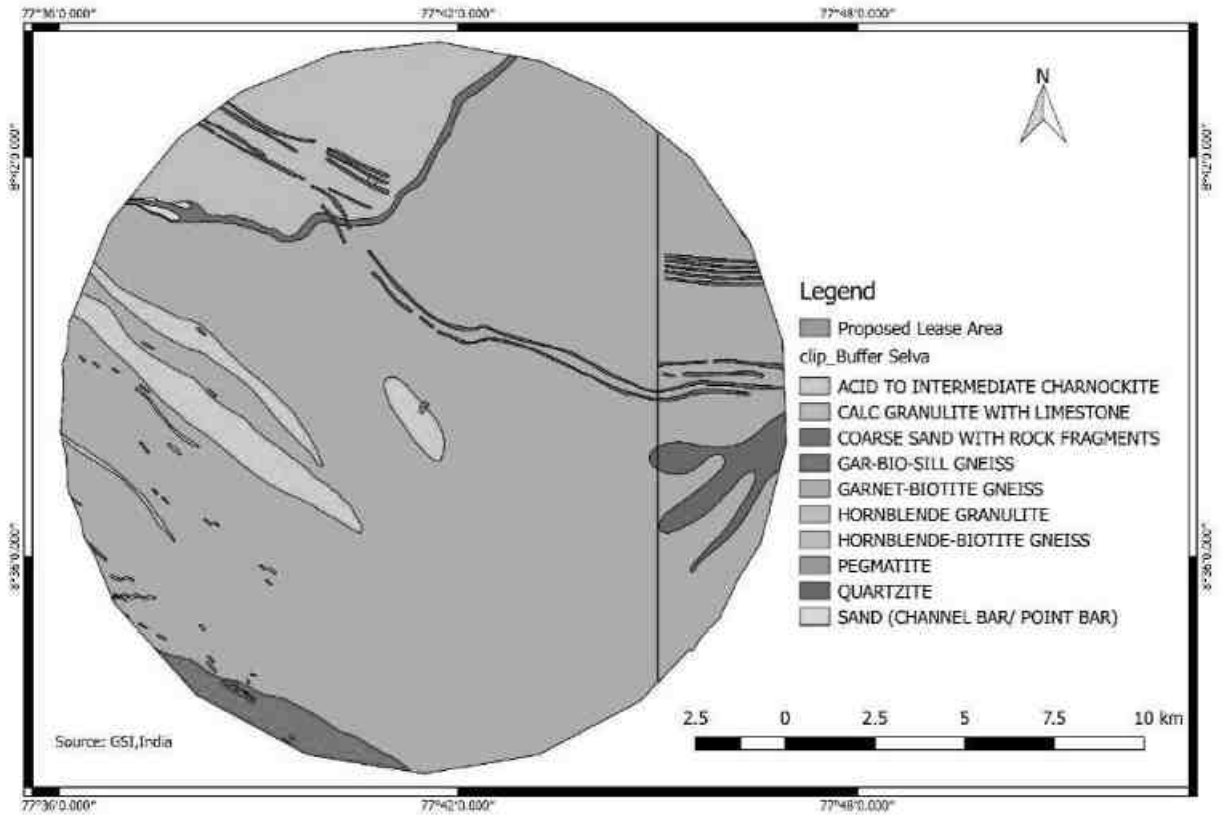
படம் 3.16 லித்தாலஜி பஃபர் மண்டல வரைபடம்
