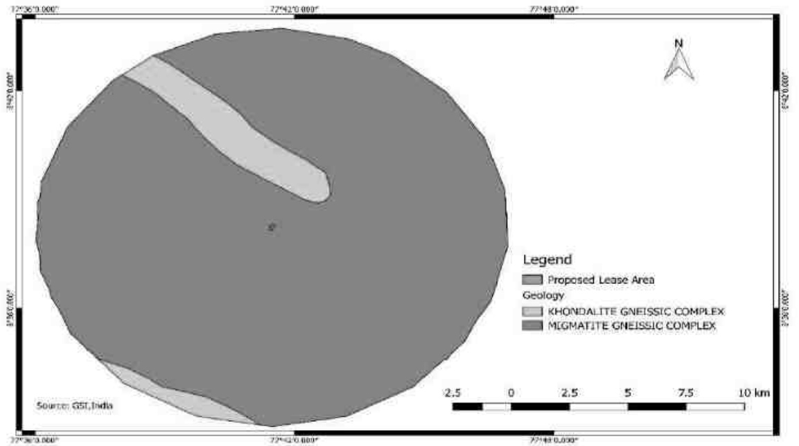
படம் 3.15 ஆய்வுப் பகுதியின் புவிபியல்
