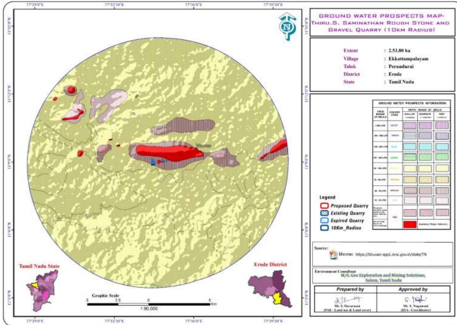
படம் 3.10: நிலத்தடி நீர் திட்ட வரைபடம்
