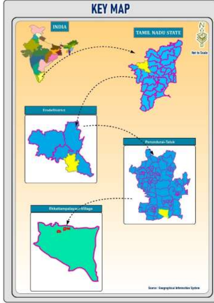
படம்1.2: திட்ட தளத்தின் இருப்பிடத்தைக் காட்டும் வரைபடம்
