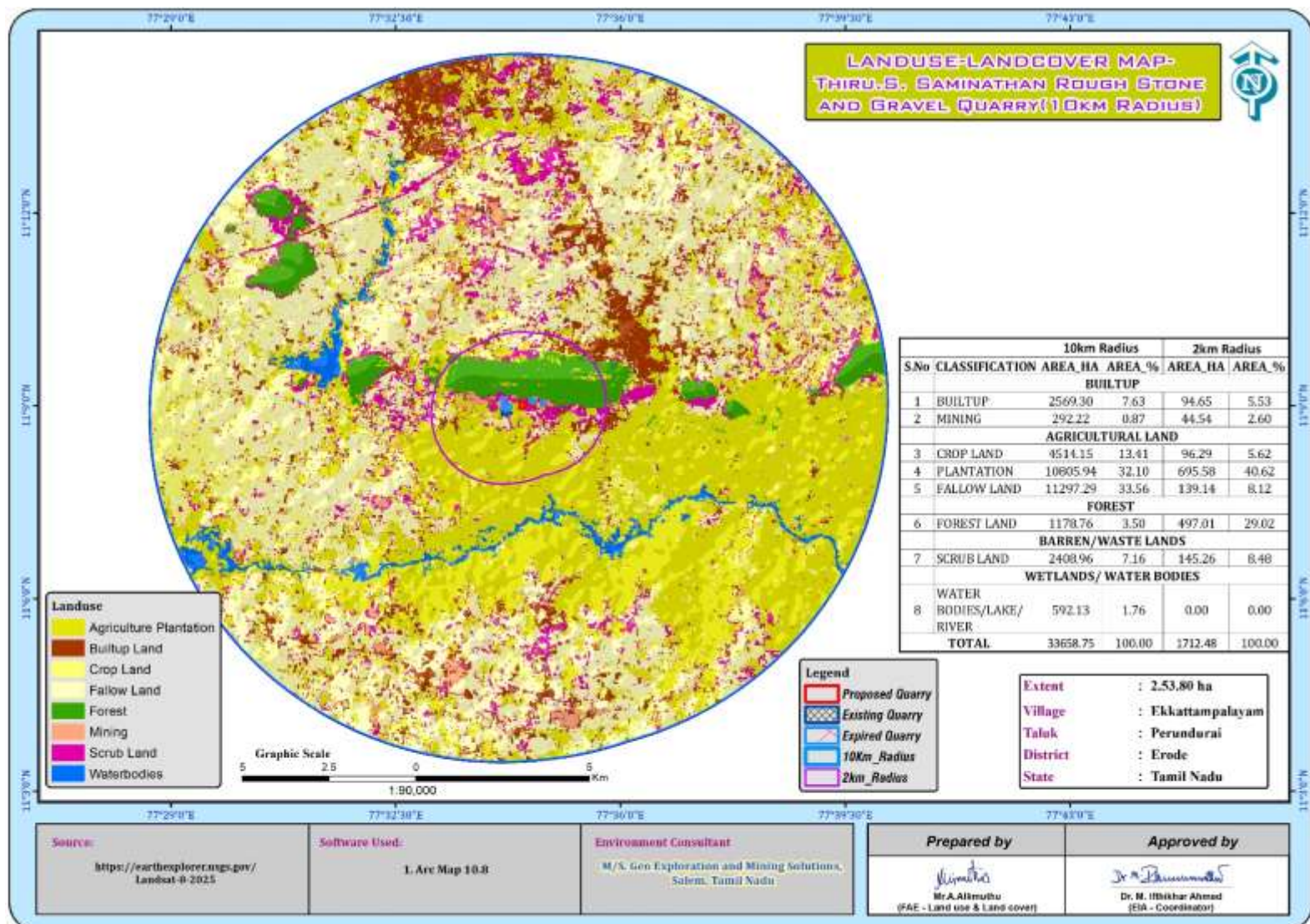
படம் 3.3: நிலப் பயன்பாடு நிலப் பரப்பு வரைபடம் 2 கி.மீ மற்றும் 10 கி.மீ சுற்றளவு
