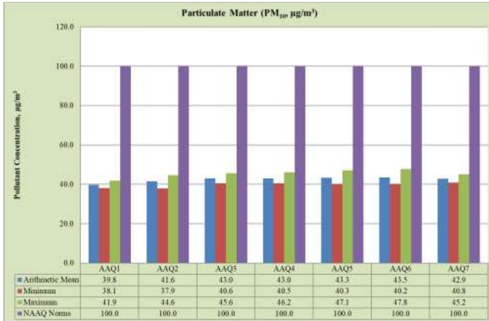
படம் 3.15: பார்டிகுலேட் மேட்டரின் பார் வரைபடம் PM 10
