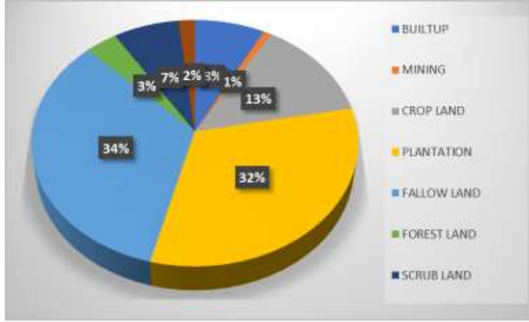
படம் 3.1: நில பயன்பாடு மற்றும் நில உறையின் பை வரைபடம் - பகுதியில் 10 கி.மீ. ஆரம்_%
