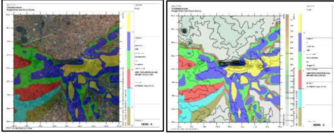
படம் 4.3: PM 2.5 இன் அதிகரிக்கும் செறிவு கணிக்கப்பட்டது
