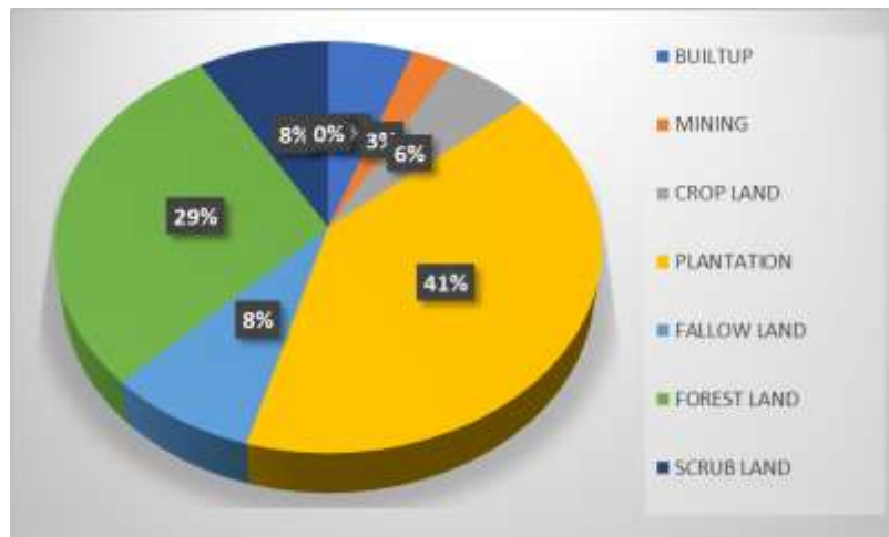
படம் 3.1-A: நில பயன்பாடு மற்றும் நில உறையின் பை வரைபடம் - பகுதியில் 2 கிமீ ஆரம்_%
