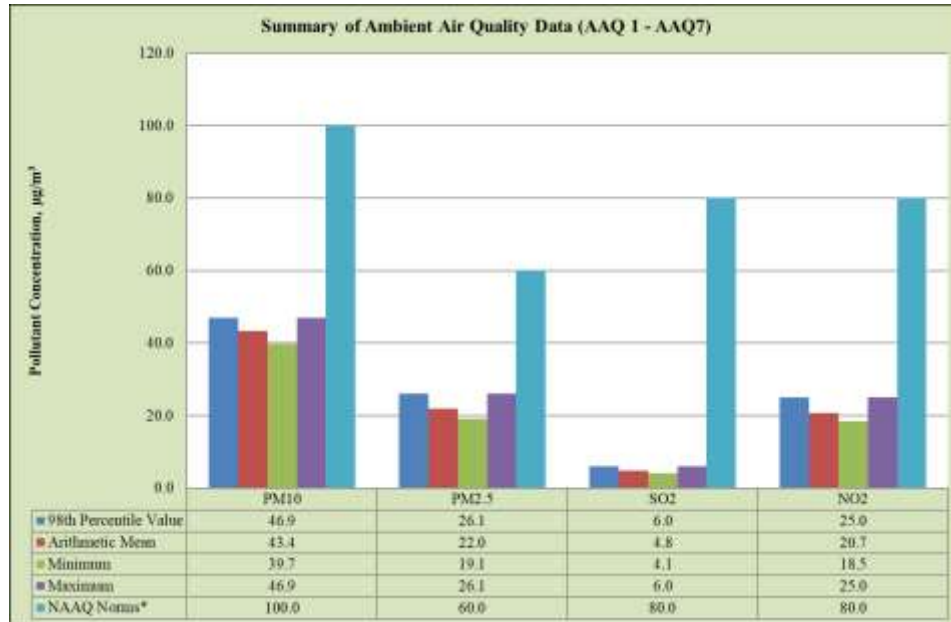
படம் 3.13: AAQ1 – AAQ7 இன் சுருக்கத்தின் பட்டி வரைபடம்
