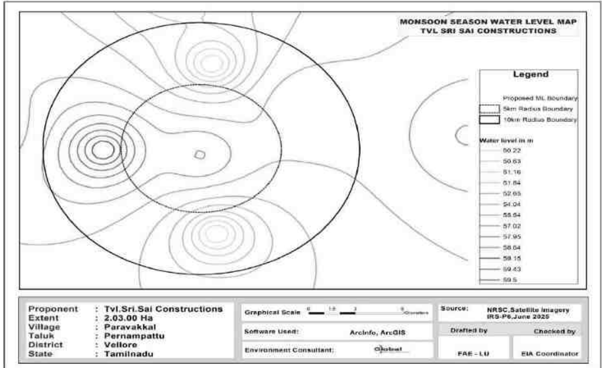
படம் 3.25 ஆய்வுப்பகுதியின்மழைக்காலநீர்நிலைவரைபடம்
