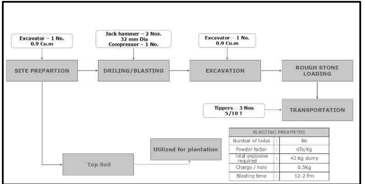
படம் 2.8 குவாரி செயல்பாட்டின் ஓட்ட விளக்கப்படம்
