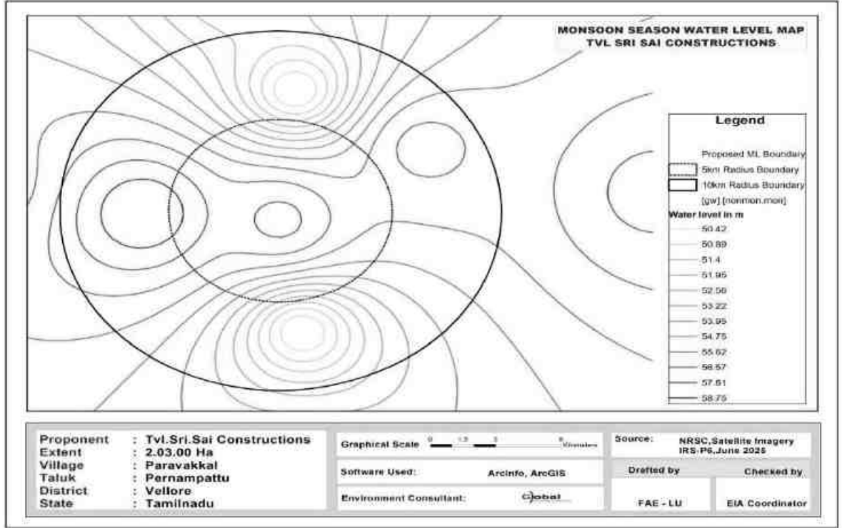
படம் 3.25 ஆய்வுப்பகுதியின்மழைக்காலநீர்நிலைவரைபடம்
