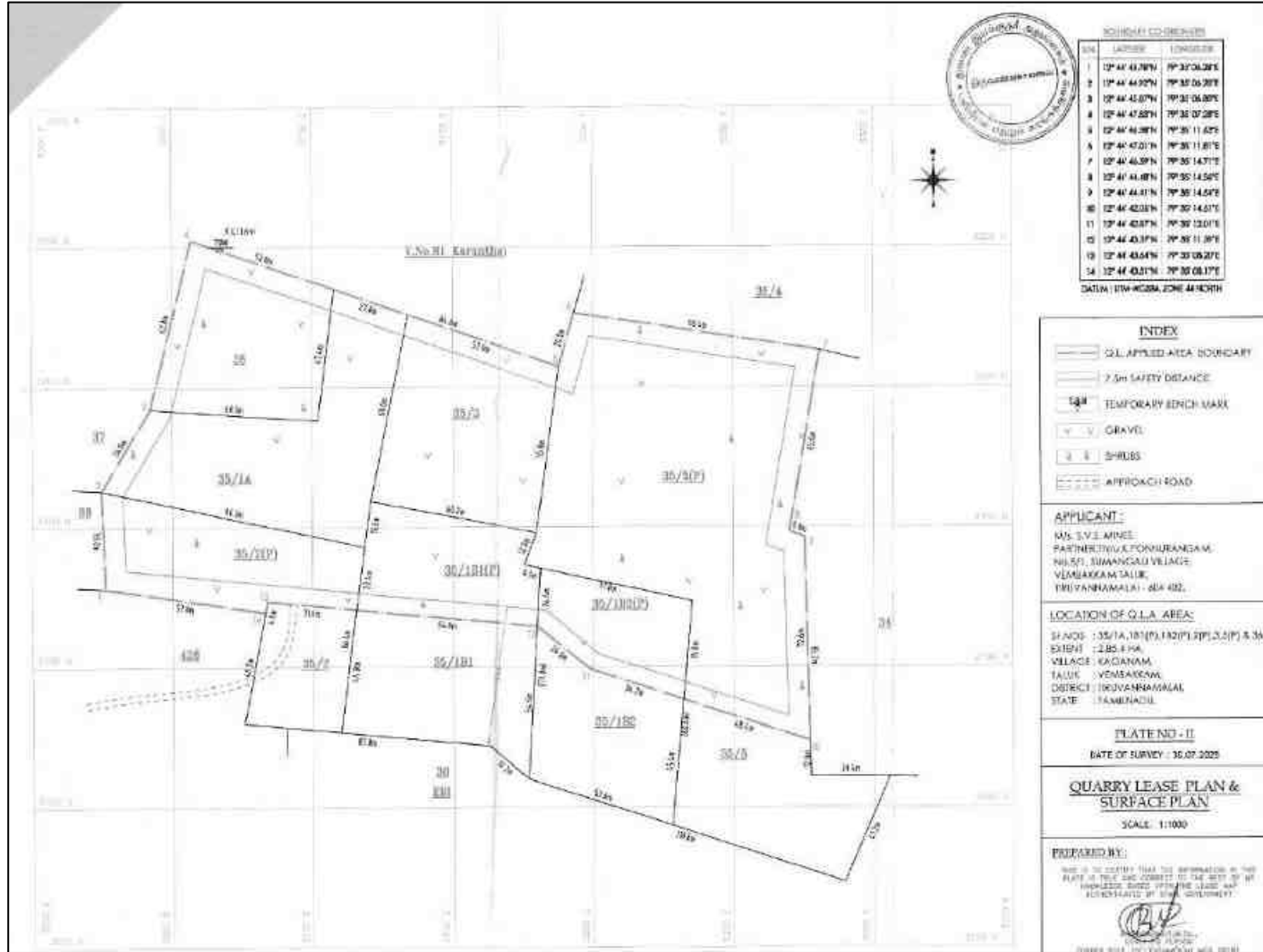
படம் 2.5: குவாரி குத்தகைத் திட்டம் / மேற்பரப்புத் திட்டம்
