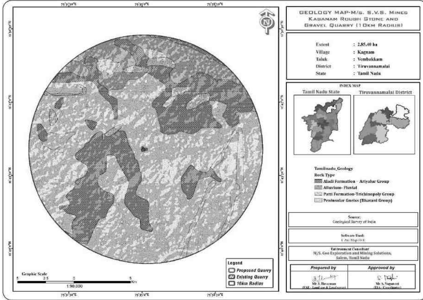
படம் 2.10 மண்டல புவிபியல் வரைபடம்
