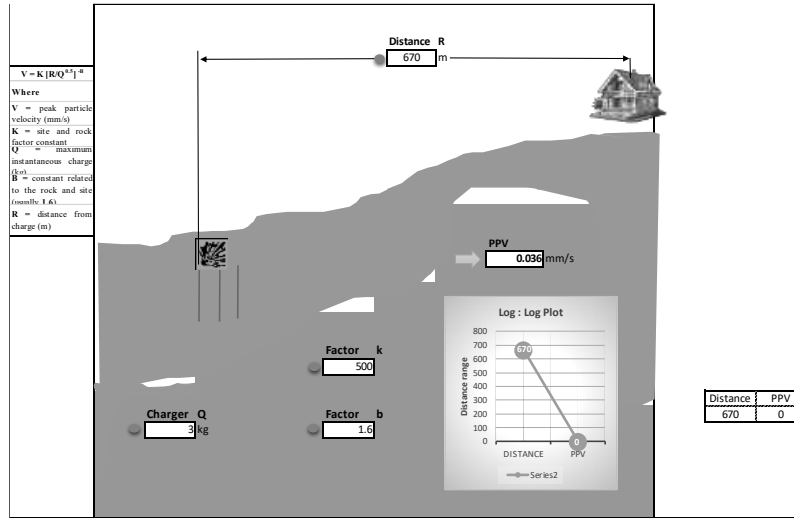
படம் 4.7: நில அதிர்வு கணிப்பு
