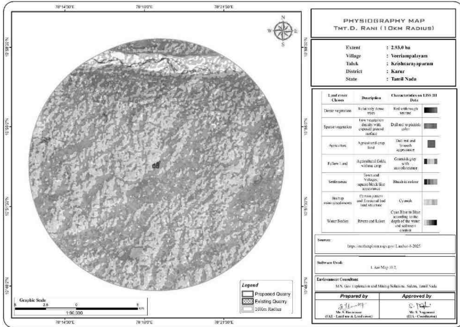
படம் 3.2: ஆய்வுப் பகுதியின் நிலவியல் வரைபடம்
