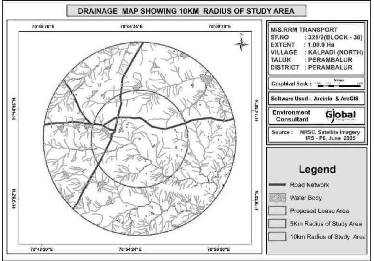
படம் 3.22 நீரோடை வடிவம் வரைபடத்தின் 10 கிலோ மீட்டர் சுற்றளவு
