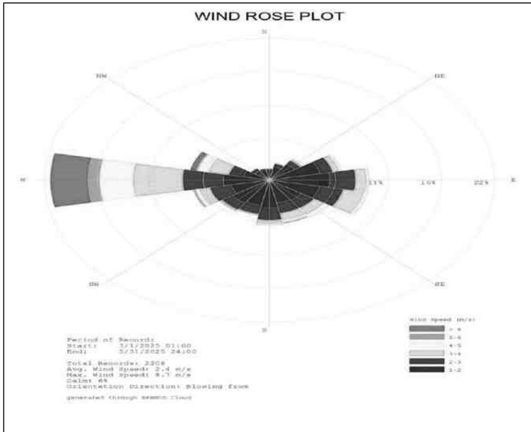
படம் 3.5 விண்ட்ரோஸ்ப்ளாட் மார்ச் 2025 இல்
