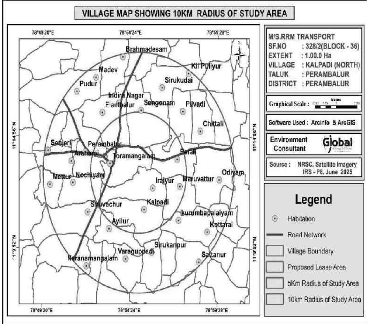
படம் 3.21 ஆய்வுப் பகுதியின் கிராம வரை படம்
