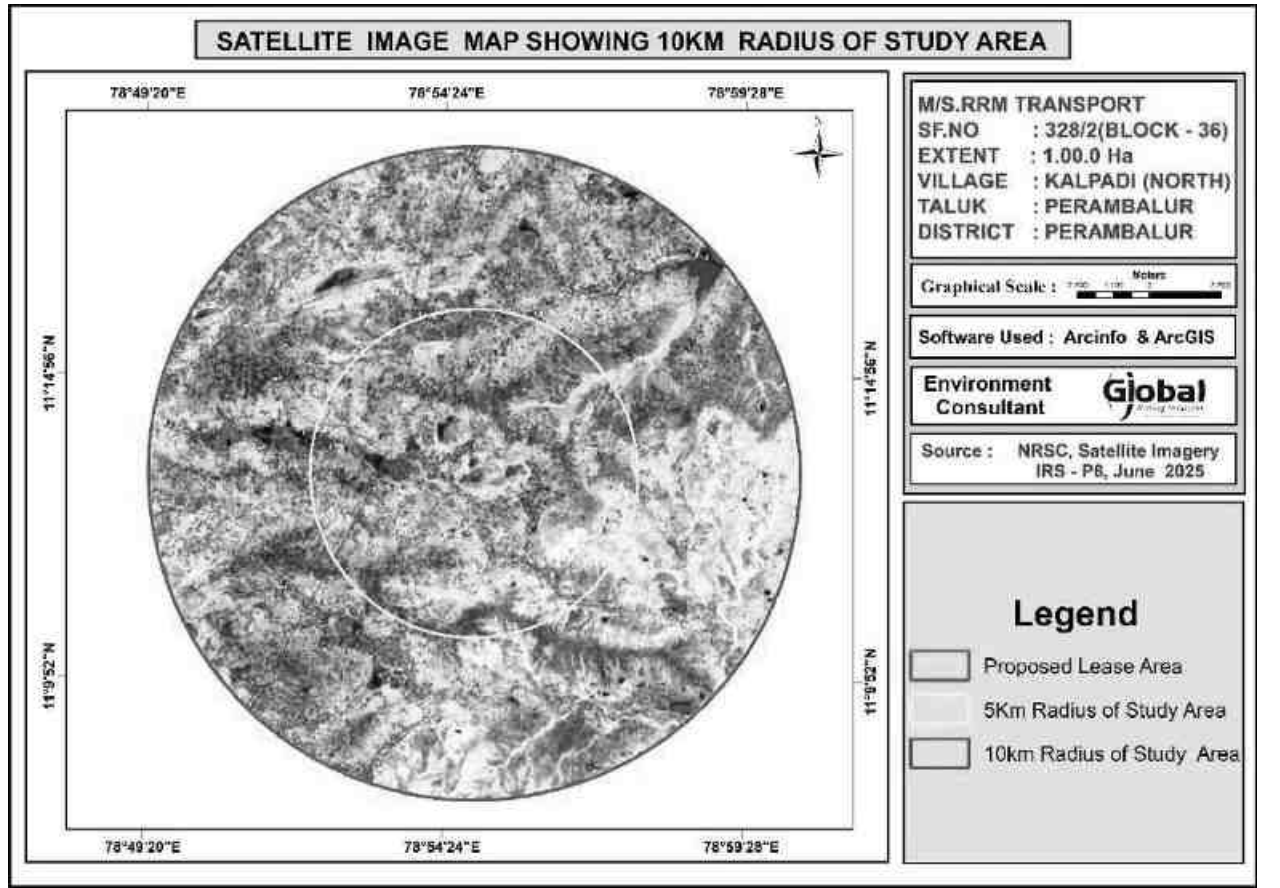
படம் எண் 3.19 தொலை உணர்வு செயற்கைக்கோள் படம்
