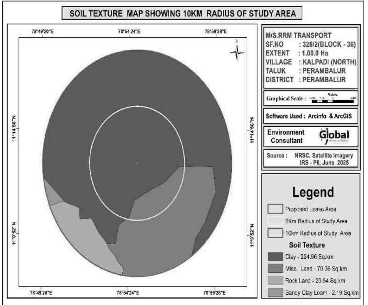
படம் 3.25 ஆய்வுப் பகுதியின் 10 கிமீ சுற்றளவு மண் வகை வரைபடம்
