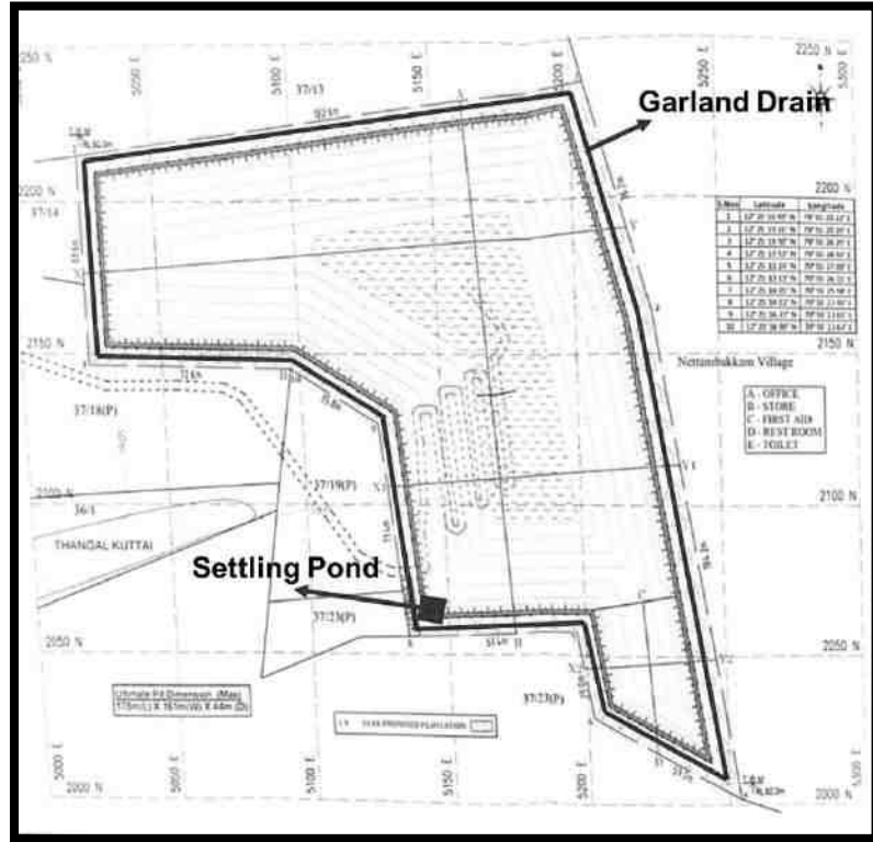
படம் 4.4: மேற்பரப்பு ஓட்ட மேலாண்மை கட்டமைப்புகள்
