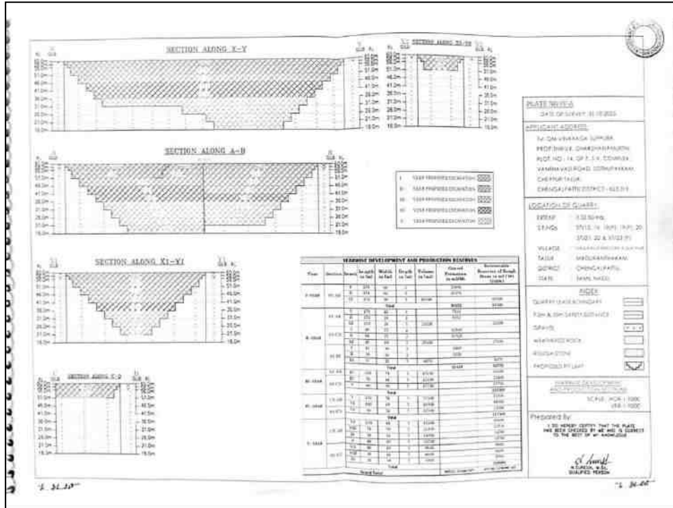
படம் 2. 11: உற்பத்தித் திட்ட குறுக்கு பிரிவு
