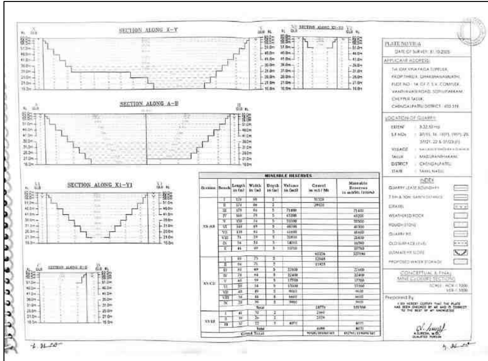
படம் 2. 13: கருத்தியல் திட்ட குறுக்கு பிரிவு
