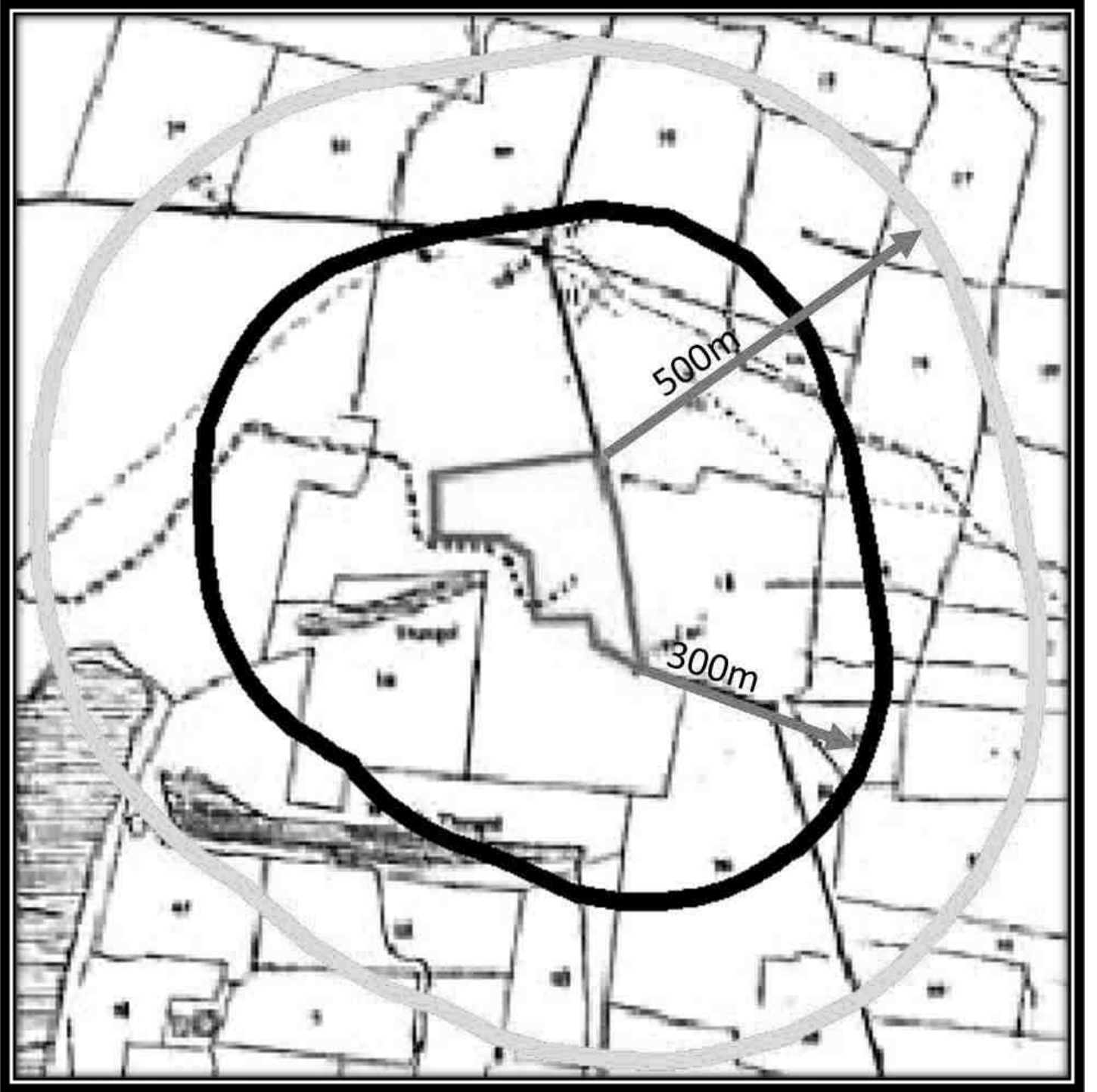
படம் 2. 5: கிராம வரைபடம்
