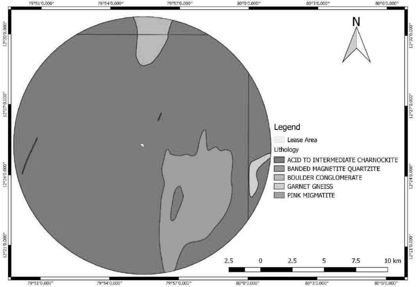
படம் 3. 21: லித்தாலஜி வரைபடம்
