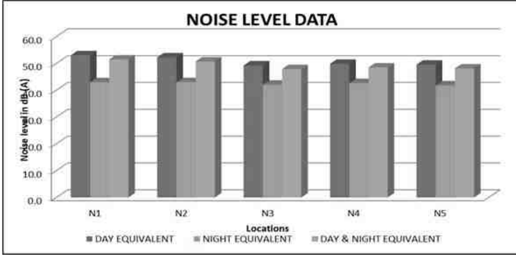
படம் 3.12:: இரைச்சல் நிலை தரவு
