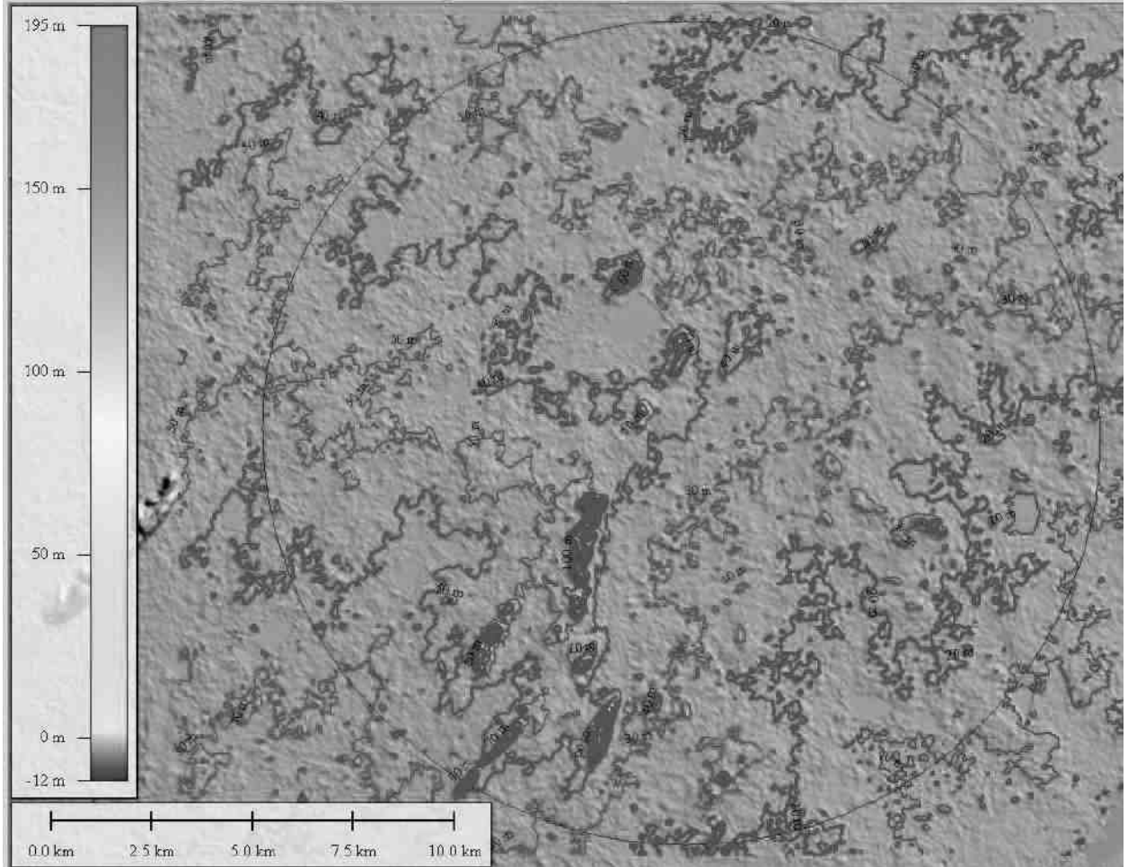
படம் 3.18: DEM வரைபடம்
