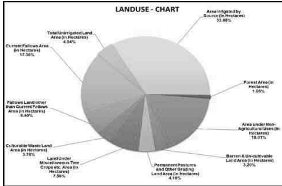
படம் 3.16: ஆய்வுப் பகுதியின் நில பயன்பாட்டு வகை .
