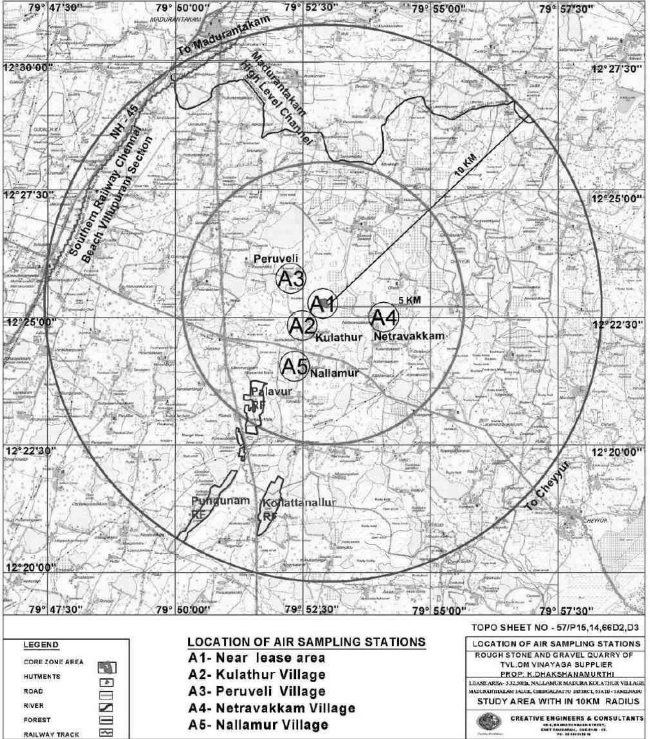
படம் 3.8: சுற்றுப்புற காற்று தர ஆய்வு நிலையங்கள்
