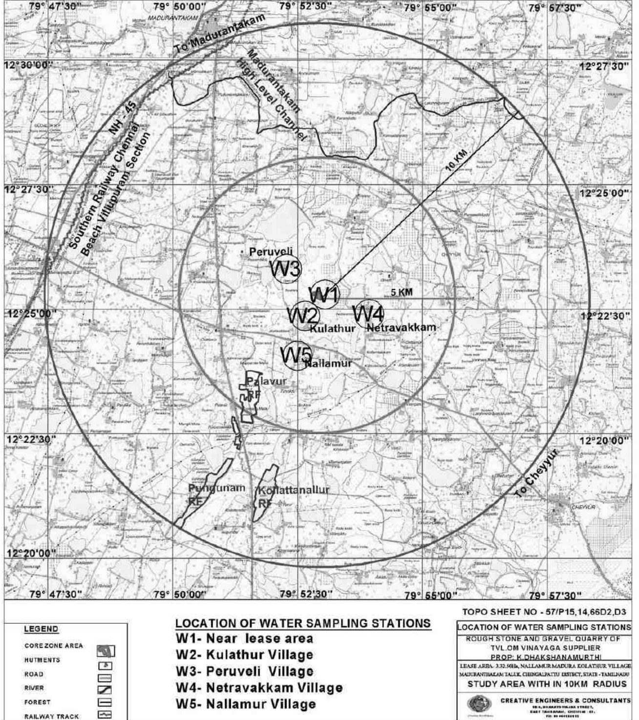
படம் 3. 10: நீர் மாதிரி நிலையங்களின் இருப்பிடம்
