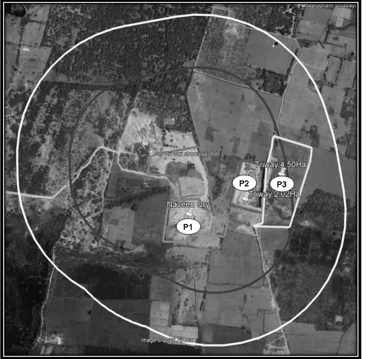
படம் 7. 1: அருகிலுள்ள குத்தகை பகுதி வரைபடம்
