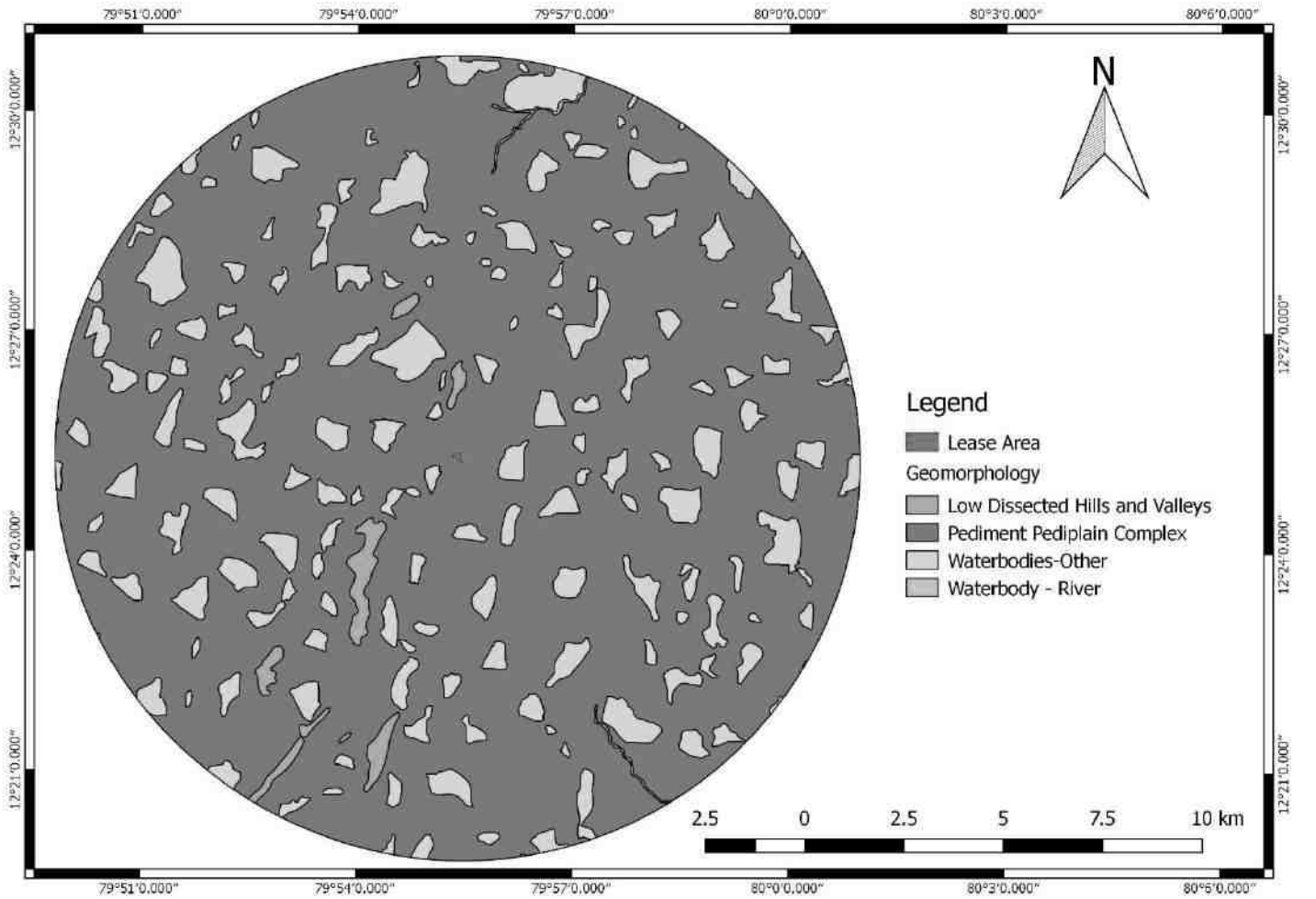
படம் 3.20: புவியியல் வரைபடம்
