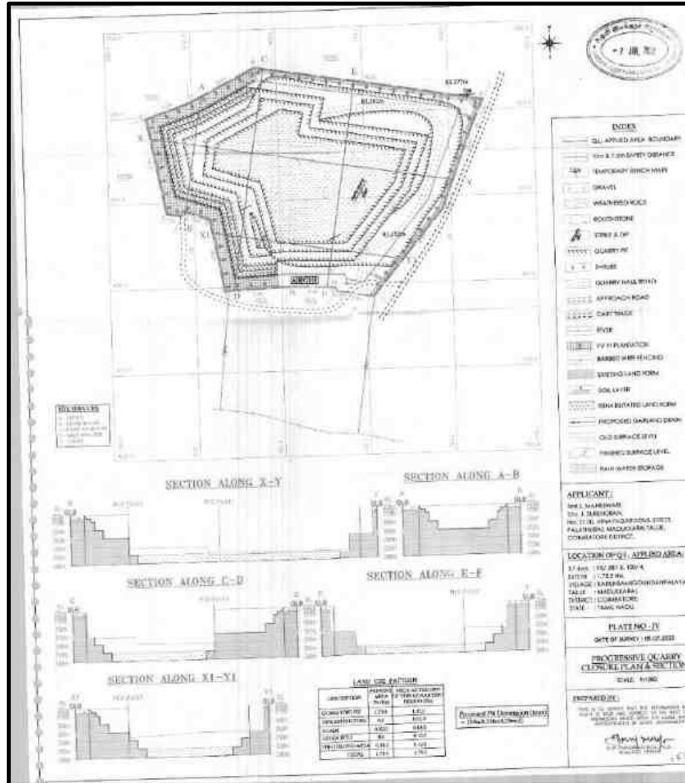
படம் 2.17: சுரங்க மூடல் திட்டம் மற்றும் பிரிவுகள் - P1
