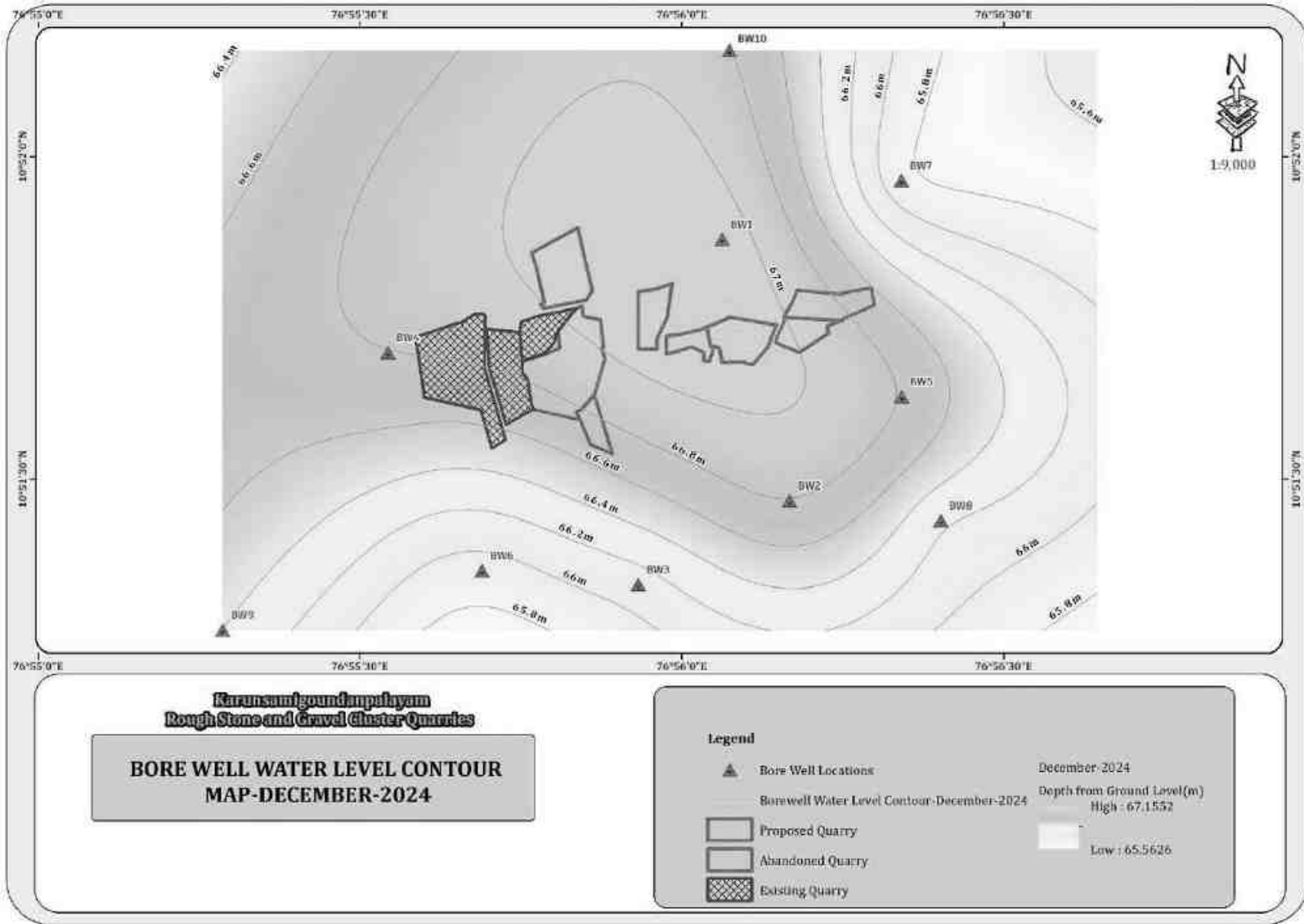
படம் 3.11: ஆழ்துளைக் கிணற்றின் மழைக்குப் பிந்தைய நீர்மட்டம் - டிசம்பர் 2024
