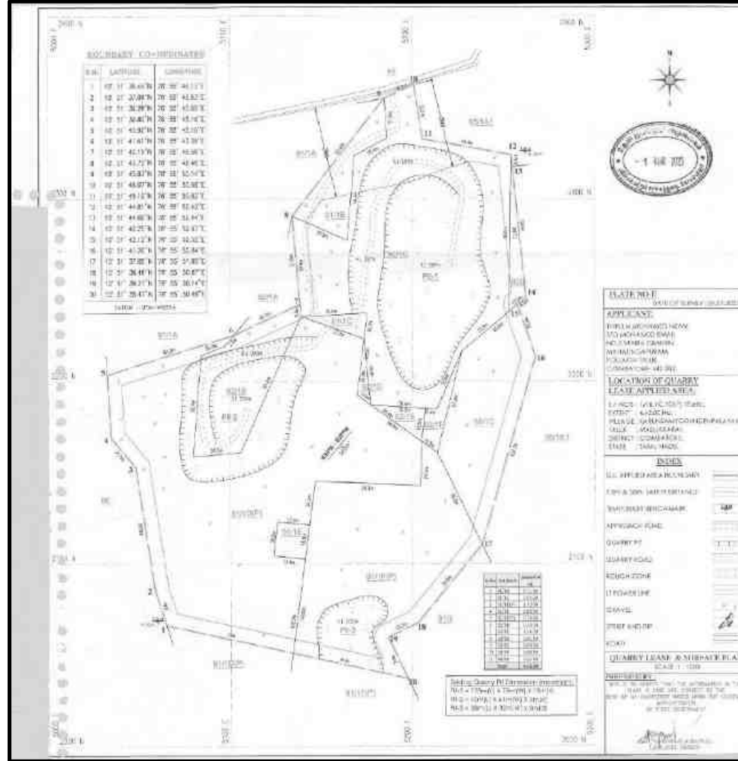
படம் 2.8: குவாரி குத்தகைத் திட்டம் / மேற்பரப்புத் திட்டம் - P2
