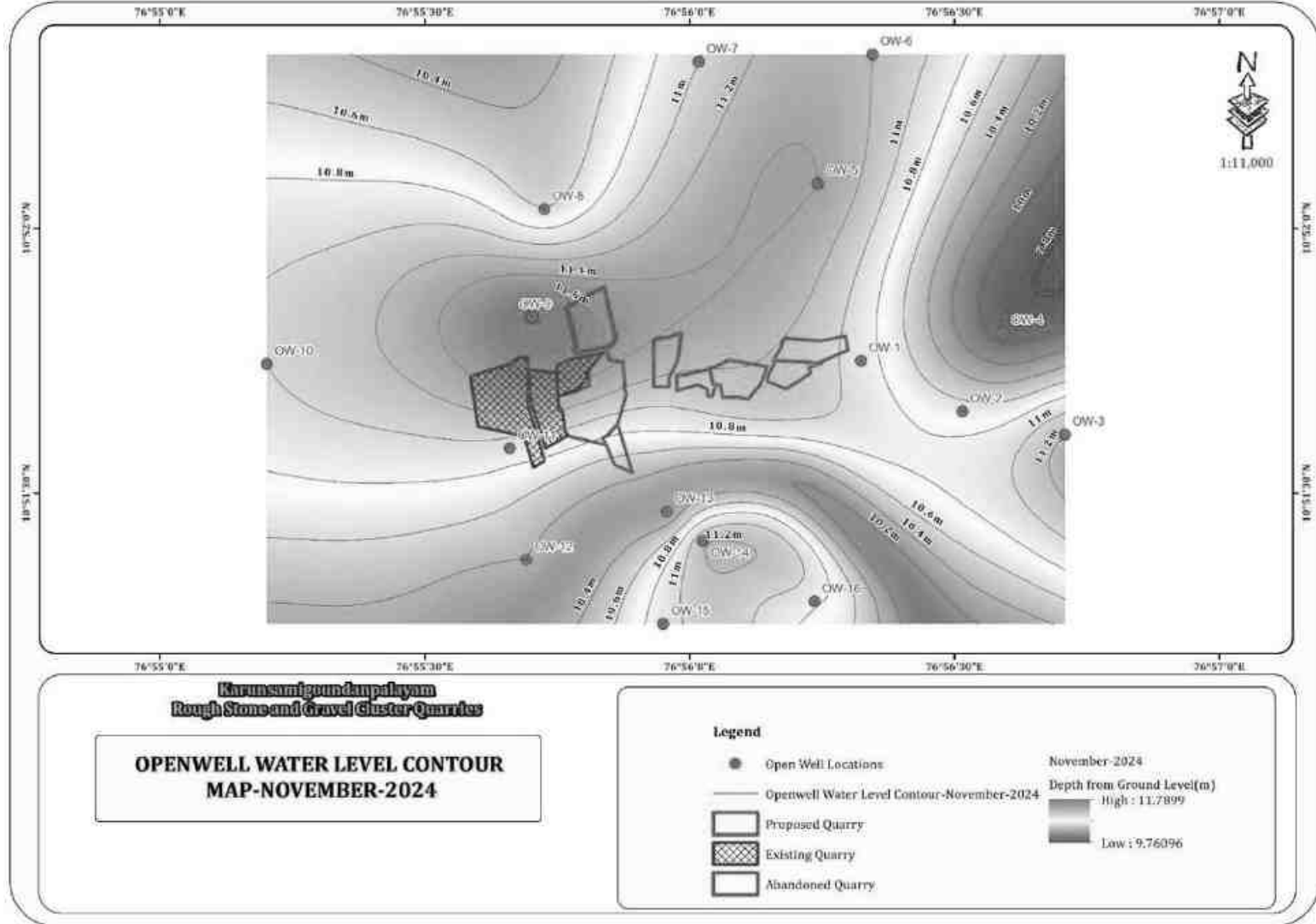
படம் 3.7: திறந்த கிணற்றின் பருவமழைக்கு பிந்தைய நீர்மட்டம் - நவம்பர் 2024
