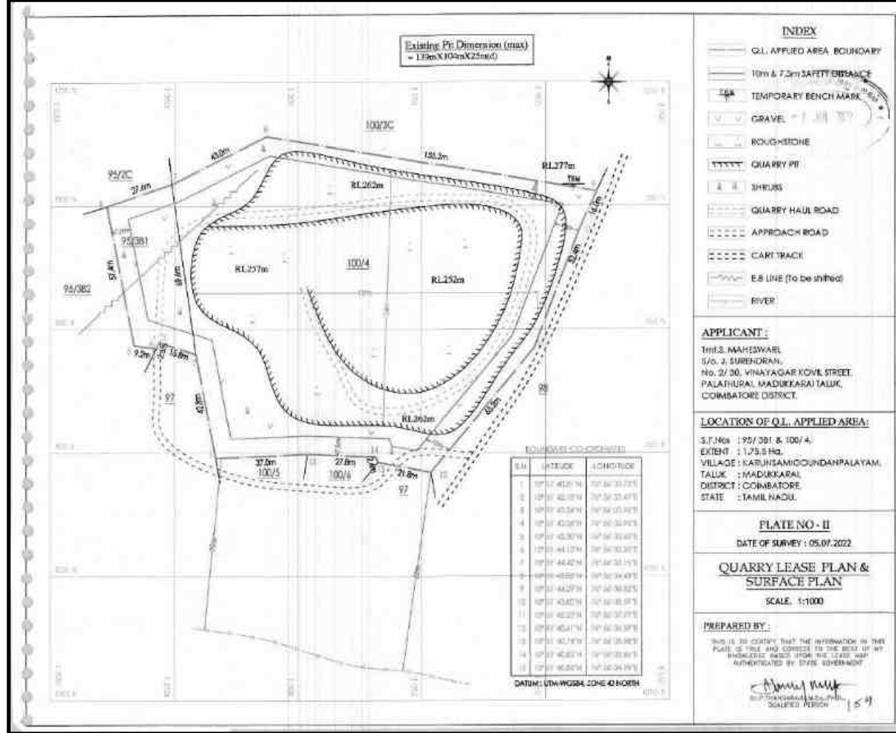
படம் 2.7: குவாரி குத்தகைத் திட்டம் / மேற்பரப்புத் திட்டம் - P1
