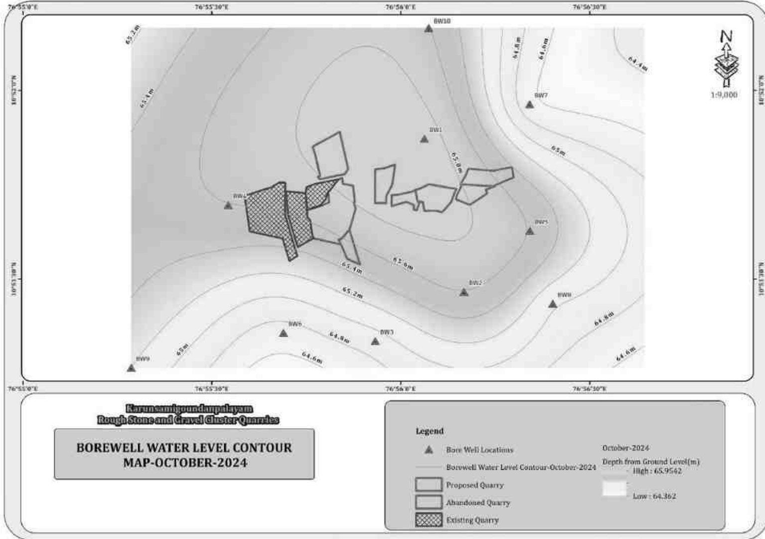
படம் 3.9: ஆழ்துளைக் கிணற்றின் மழைக்குப் பிந்தைய நீர்மட்டம் - அக்டோபர் 2024
