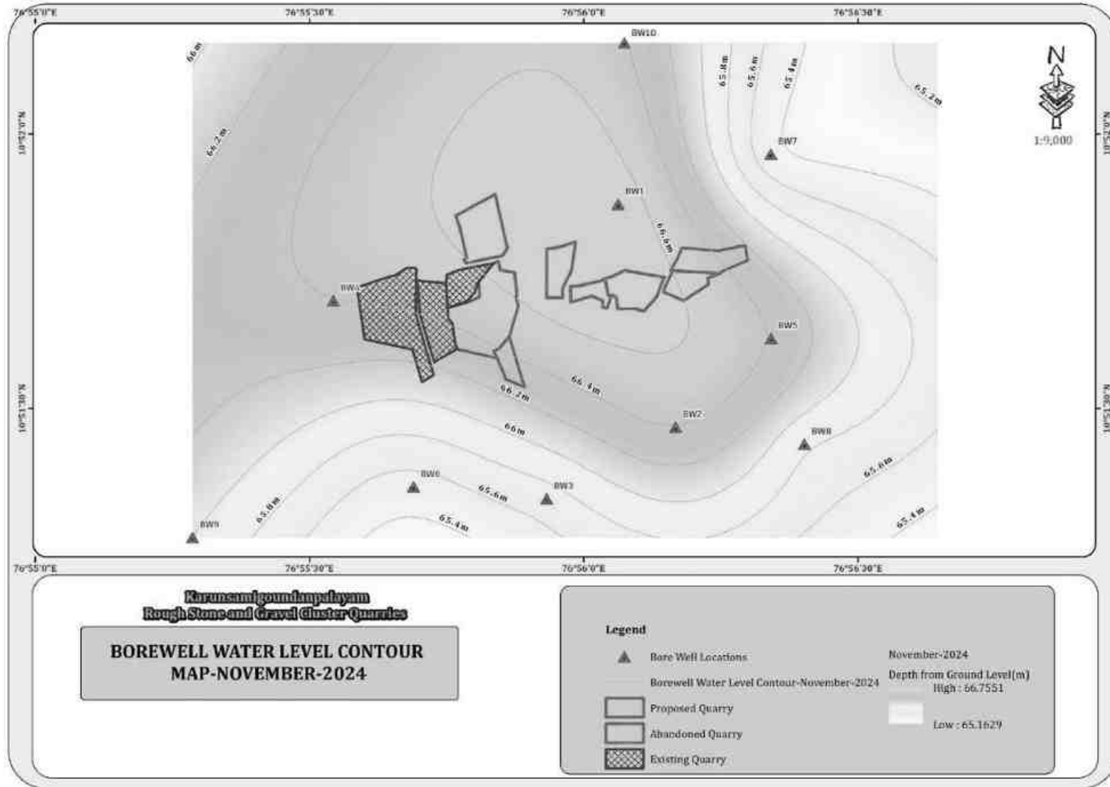
படம் 3.10: ஆழ்துளைக் கிணற்றின் மழைக்குப் பிந்தைய நீர்மட்டம் - நவம்பர் 2024
