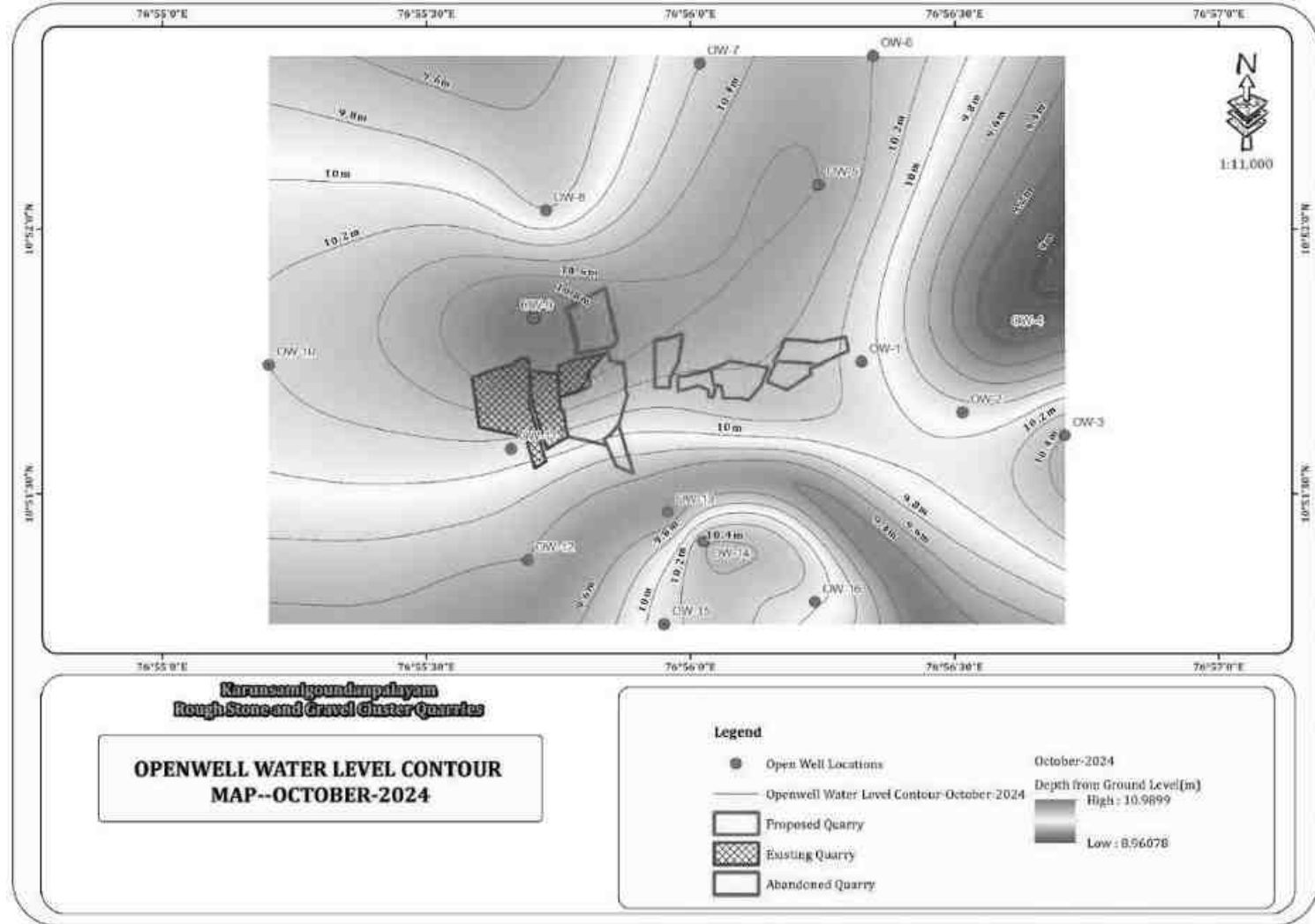
படம் 3.6: திறந்த கிணற்றின் பருவமழைக்கு பிந்தைய நீர்மட்டம் - அக்டோபர் 2024
