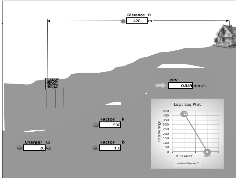
படம் 4.7: நில அதிர்வு கணிப்பு - P2
