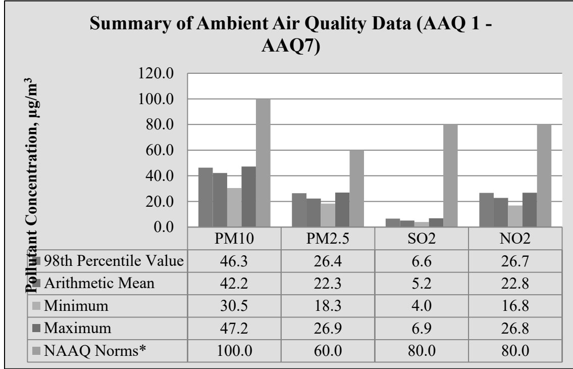
படம் 3.13: காற்றின் தர மாதிரியின் சுருக்க வரைபடம் (AAQ1-AAQ7)
