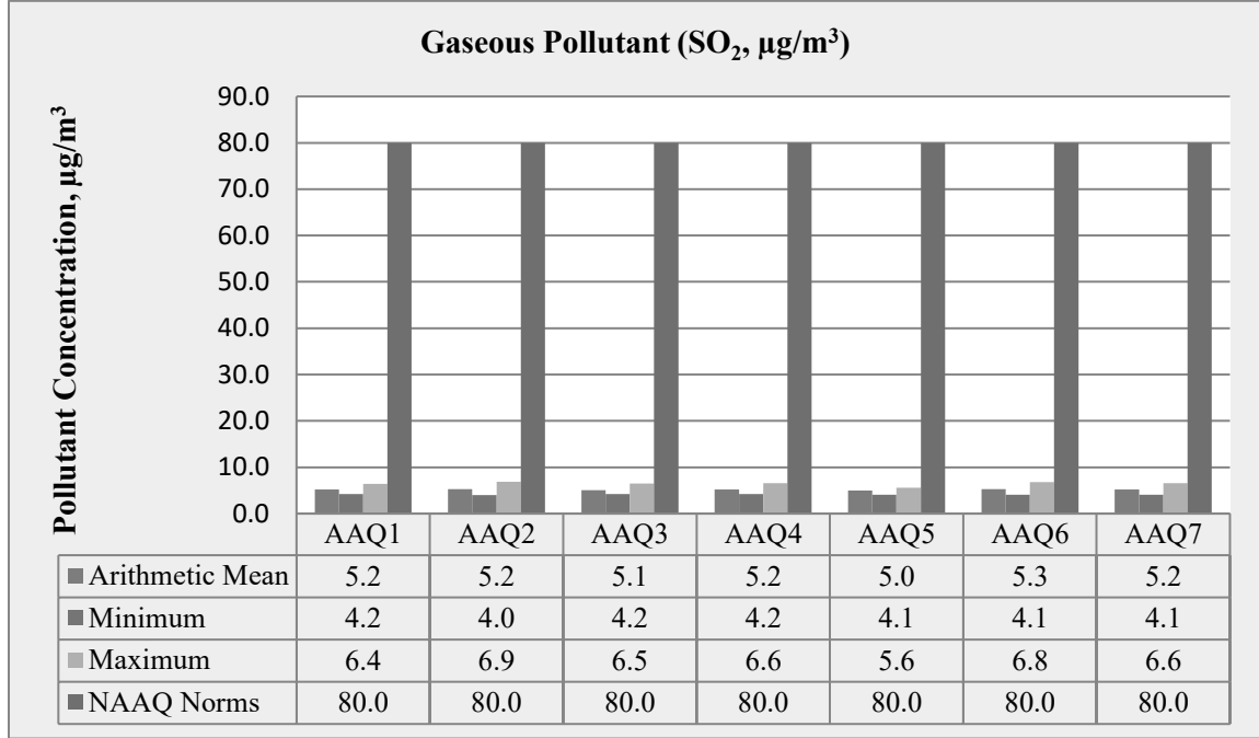
படம் 3.19: காற்றின் தர மாதிரியின் சுருக்க வரைபடம் SO 2
