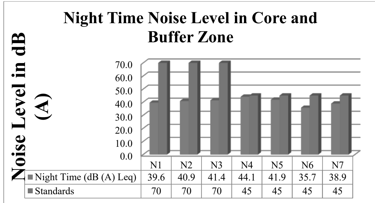
படம் 3.20: மைய மற்றும் இடையக மண்டலத்தில் இரவு நேர இரைச்சல் நிலைகள்
