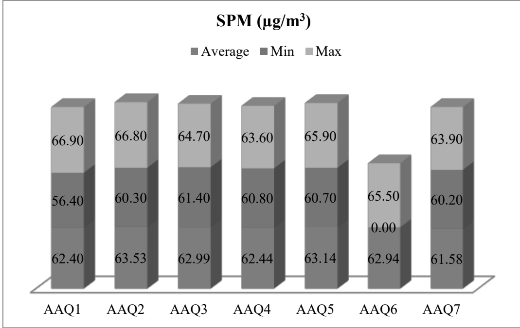
படம் 3.18: SPM மதிப்புகளின் பட்டை வரைபடம்
