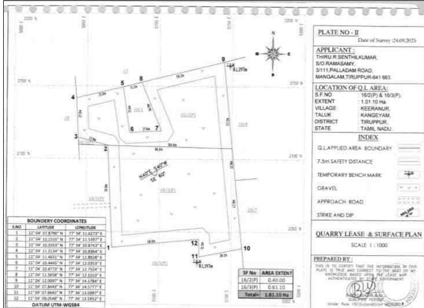
படம் 2.4: குவாரி குத்தகைத் திட்டம் / மேற்பரப்புத் திட்டம் - P1
