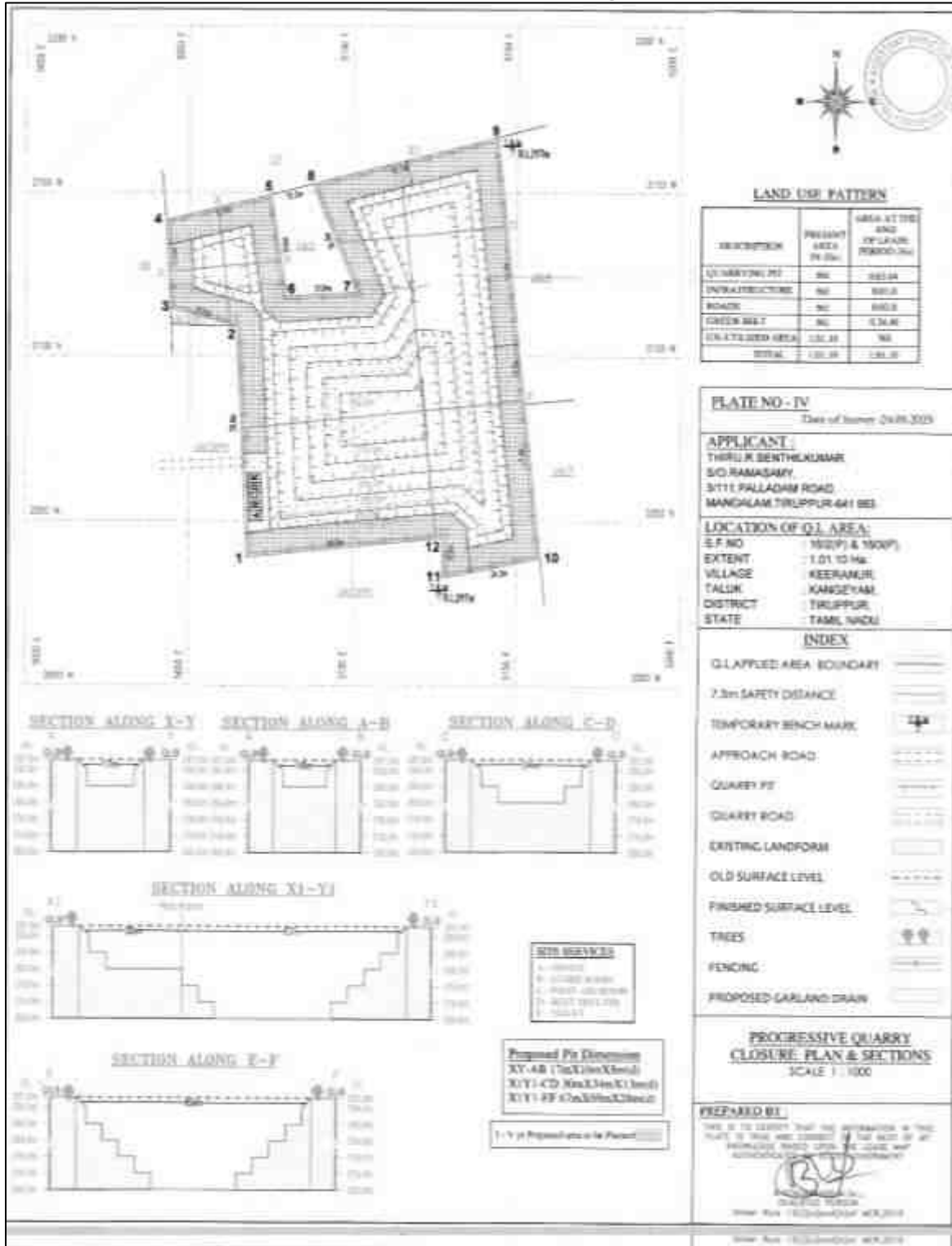
படம் 2.11: சுரங்க மூடல் வரைபடம் மற்றும் பிரிவுகள் - P1
