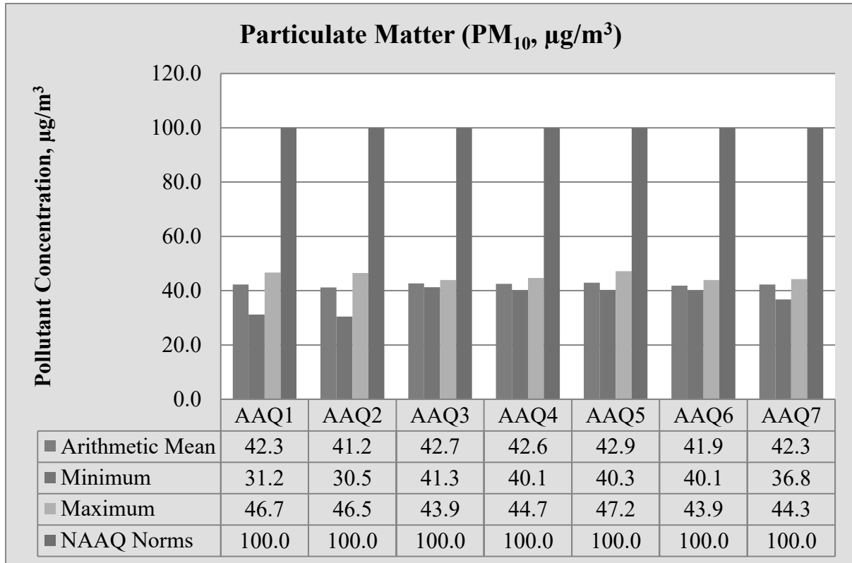
படம் 3.15: காற்றின் தர மாதிரியின் சுருக்க வரைபடம் PM 10
