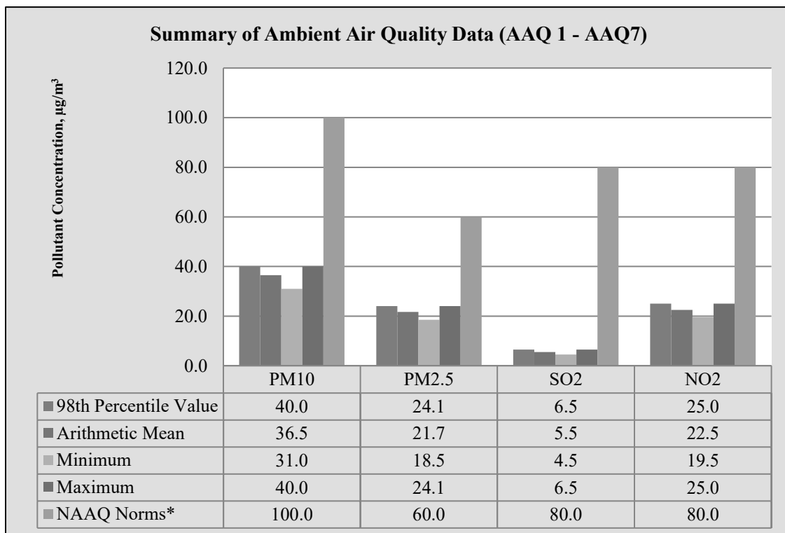
படம் 3.14: AAQ1 – AAQ7 இன் சுருக்கத்தின் பட்டி வரைபடம்
