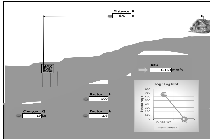
படம் 4.6: நில அதிர்வு கணிப்பு
