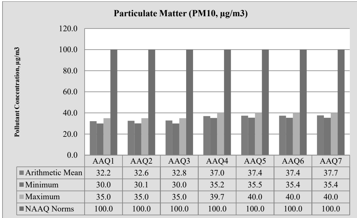
படம் 3.16: பார்டிகுலேட் மேட்டரின் பார் வரைபடம் PM 10
