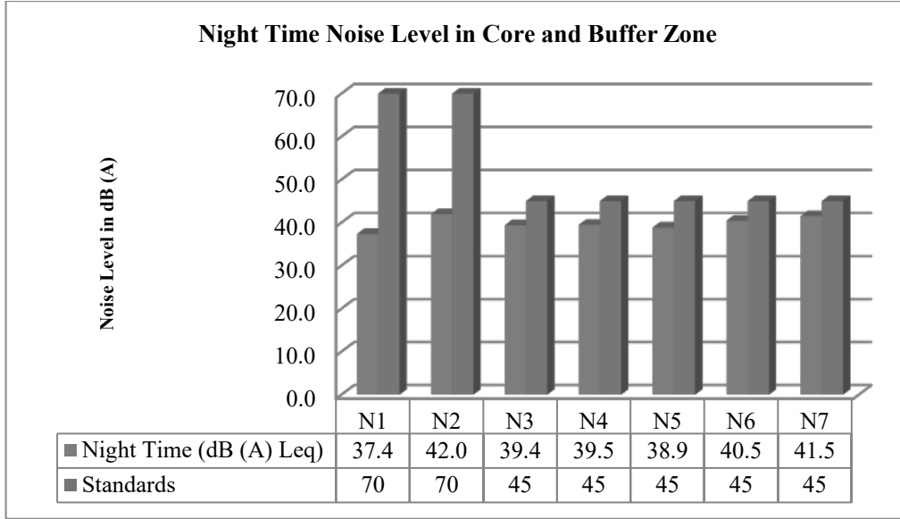
படம் 3.23: முக்கிய மற்றும் இடையக மண்டலத்தில் இரவு நேர இரைச்சல் நிலைகள்
