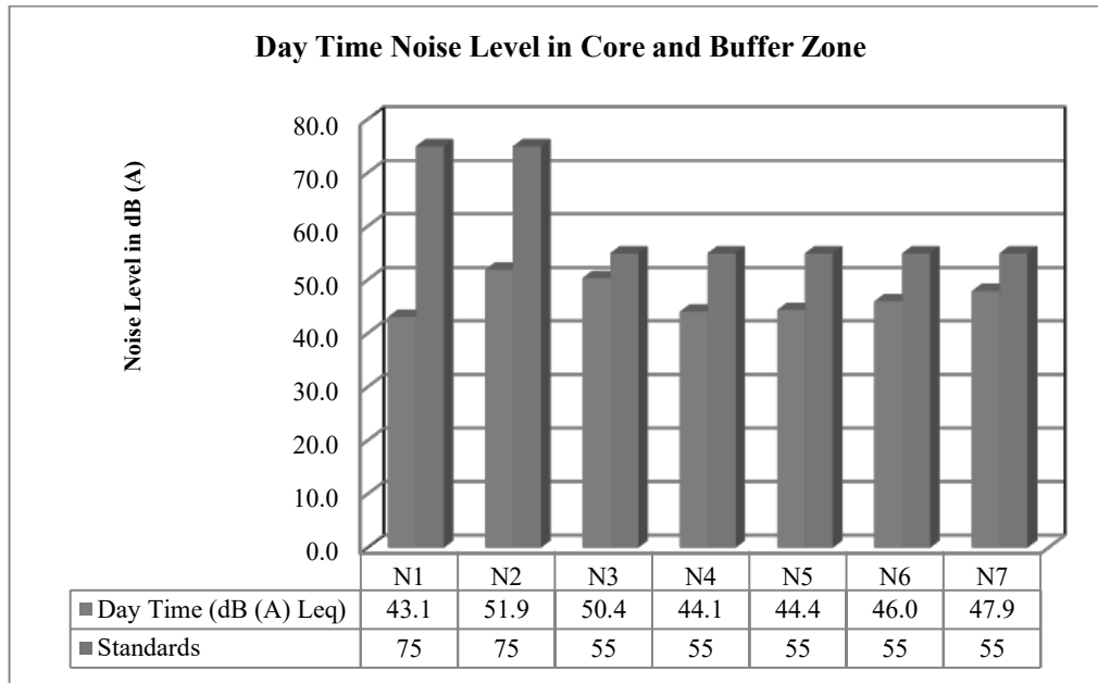
படம் 3.22: முக்கிய மற்றும் இடையக மண்டலத்தில் பகல் நேர இரைச்சல் நிலைகள்
