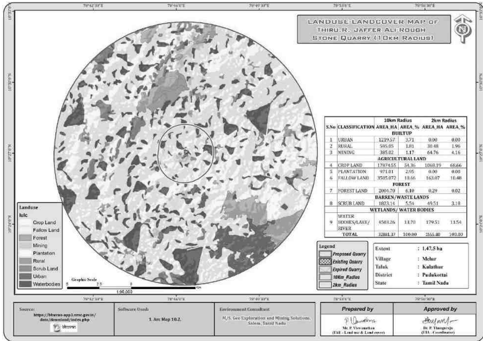
படம் 3.2: நில பயன்பாட்டு வரைபடம் 2 கி.மீ மற்றும் 10 கி.மீ சுற்றளவு
