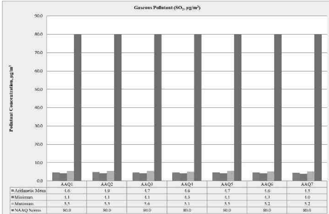
படம் 3.14: காற்றின் தர மாதிரியின் சுருக்க வரைபடம் SO 2
