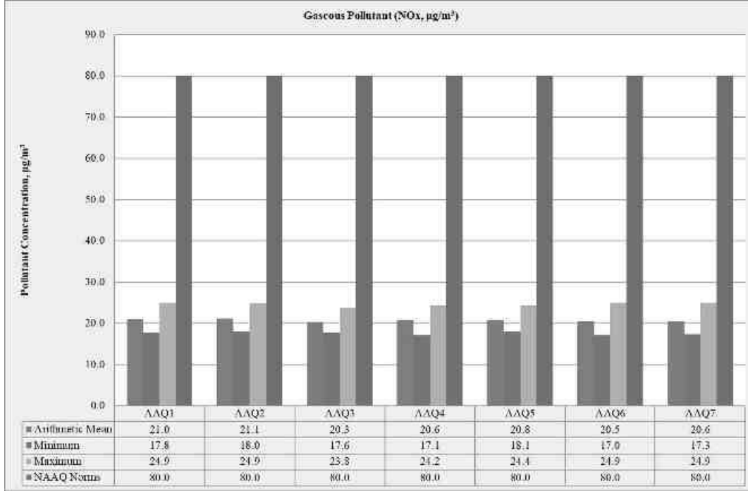
படம் 3.15: காற்றின் தர மாதிரியின் சுருக்க வரைபடம் NO x
