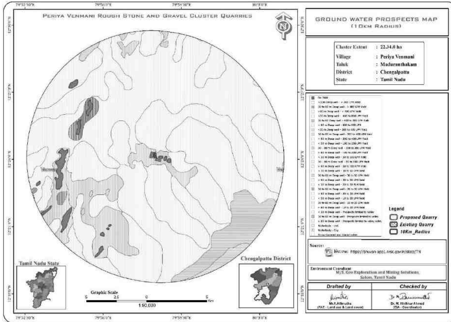
படம் 3.11: நிலத்தடி நீர் திட்ட வரைபடம்
