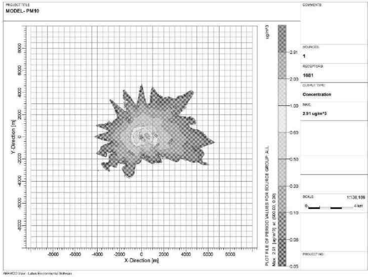
படம் 4.3 - PM10 க்கான GLC கணிப்பின் ஐசோப்லெத்
