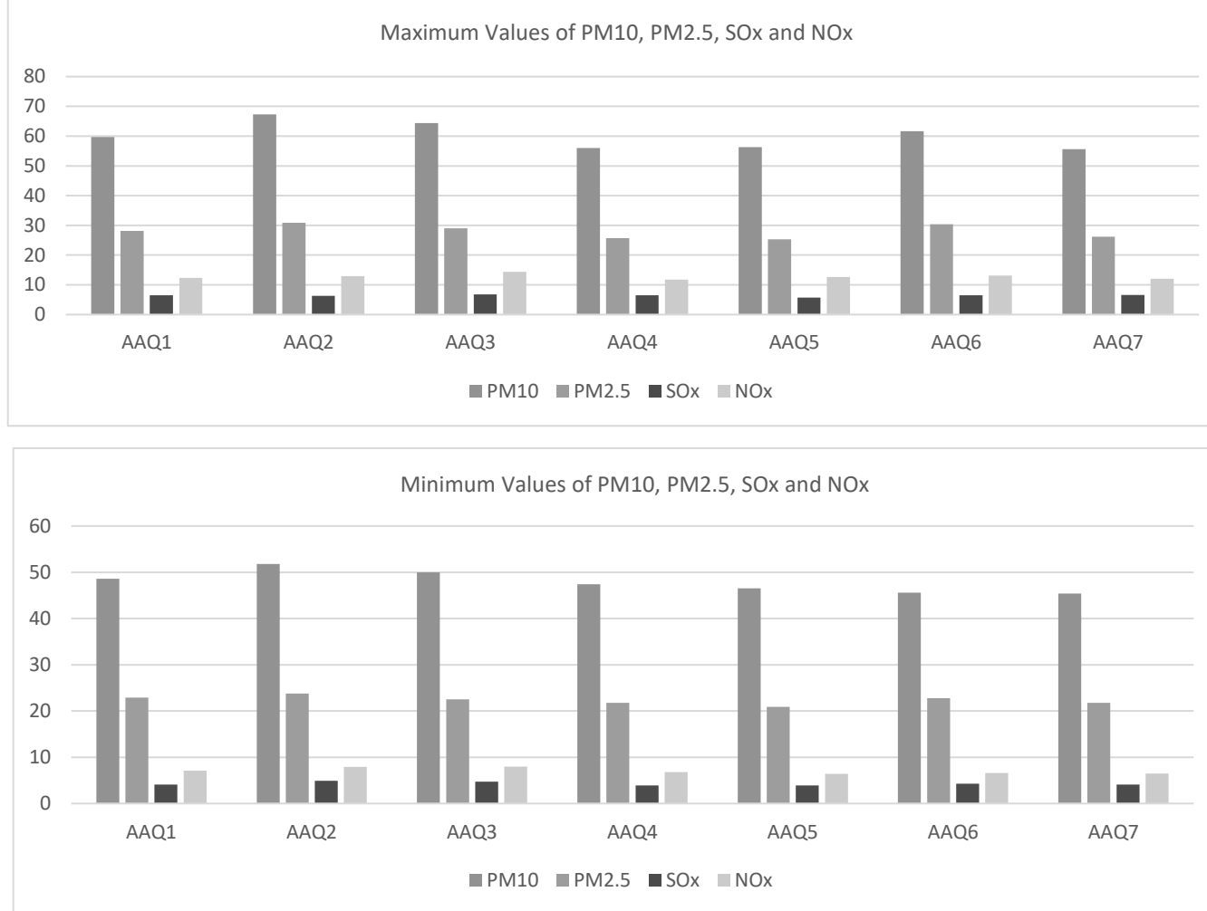
படம் - 3.9 - காற்றின் தர தரவுகளின் வரைகலை பிரதிநிதித்துவம்
