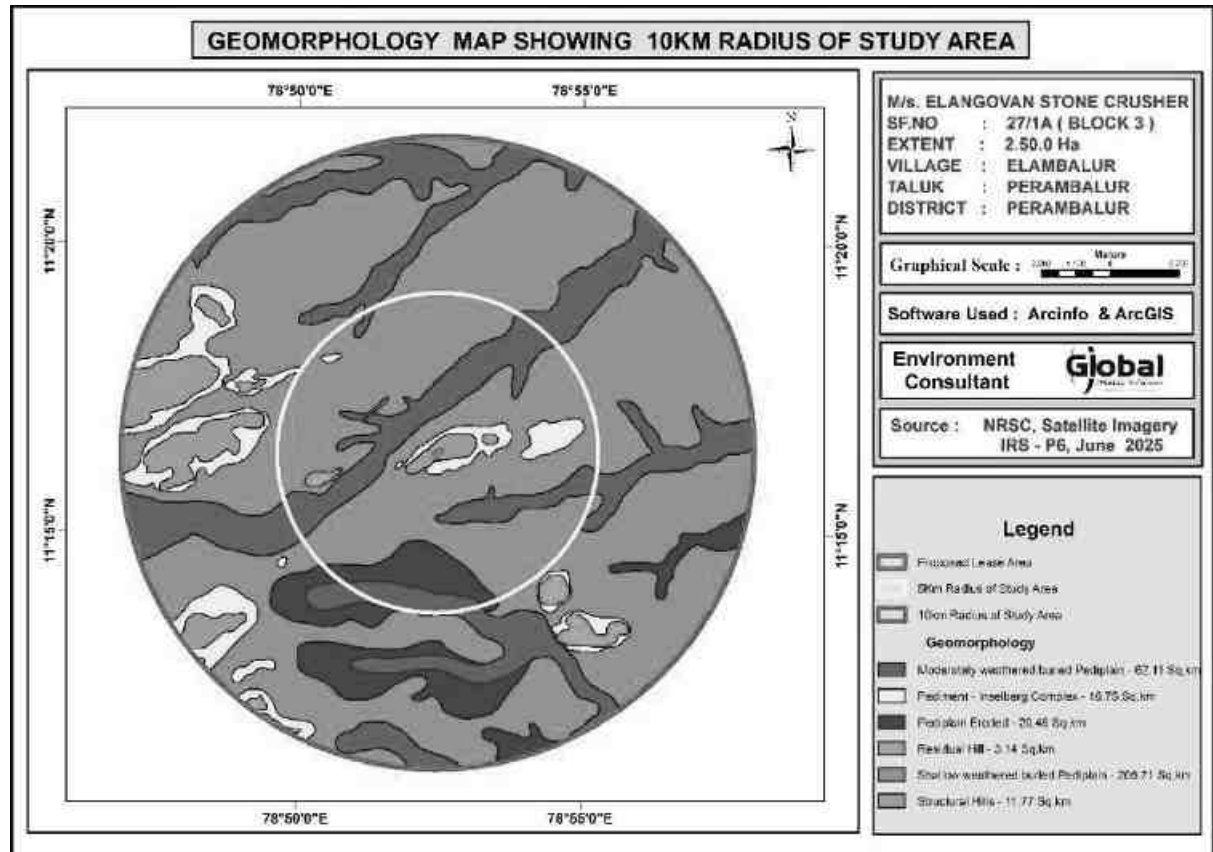
படம் 3.17 ஆய்வுப் பகுதியின் புவி உருவவியல் வரைபடம்
