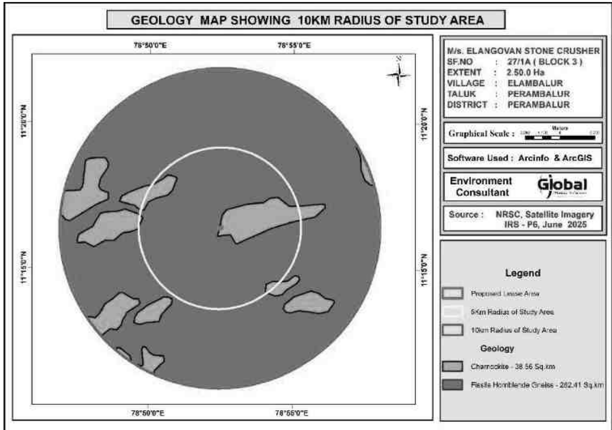
படம் 3.18 ஆய்வுப் பகுதியின் புவியியல் வரைபடம்
