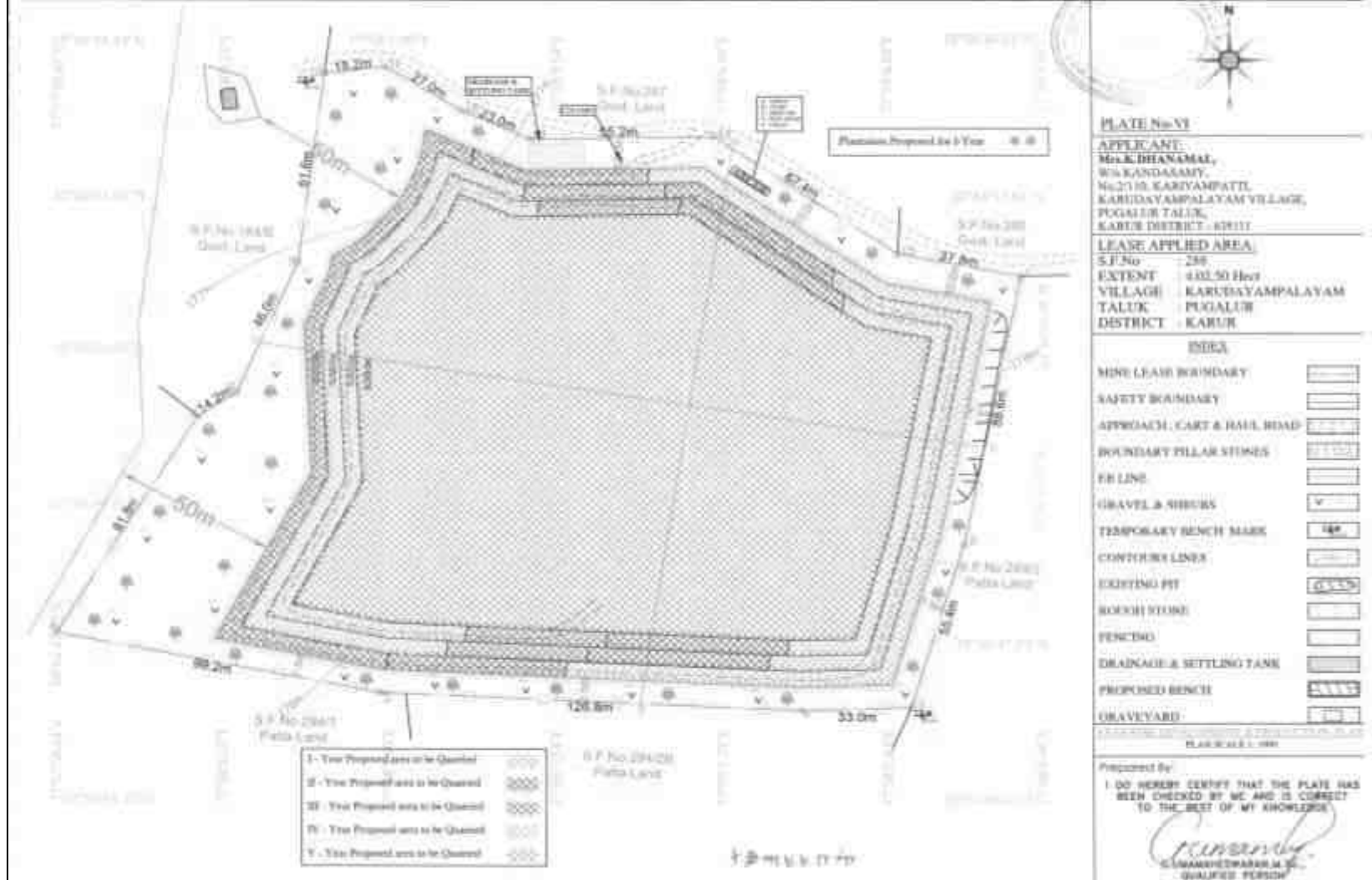
படம் 2.4 ஆண்டு வாரியான உற்பத்தித் திட்டம் & பிரிவு (ஐந்து ஆண்டுகள்)
