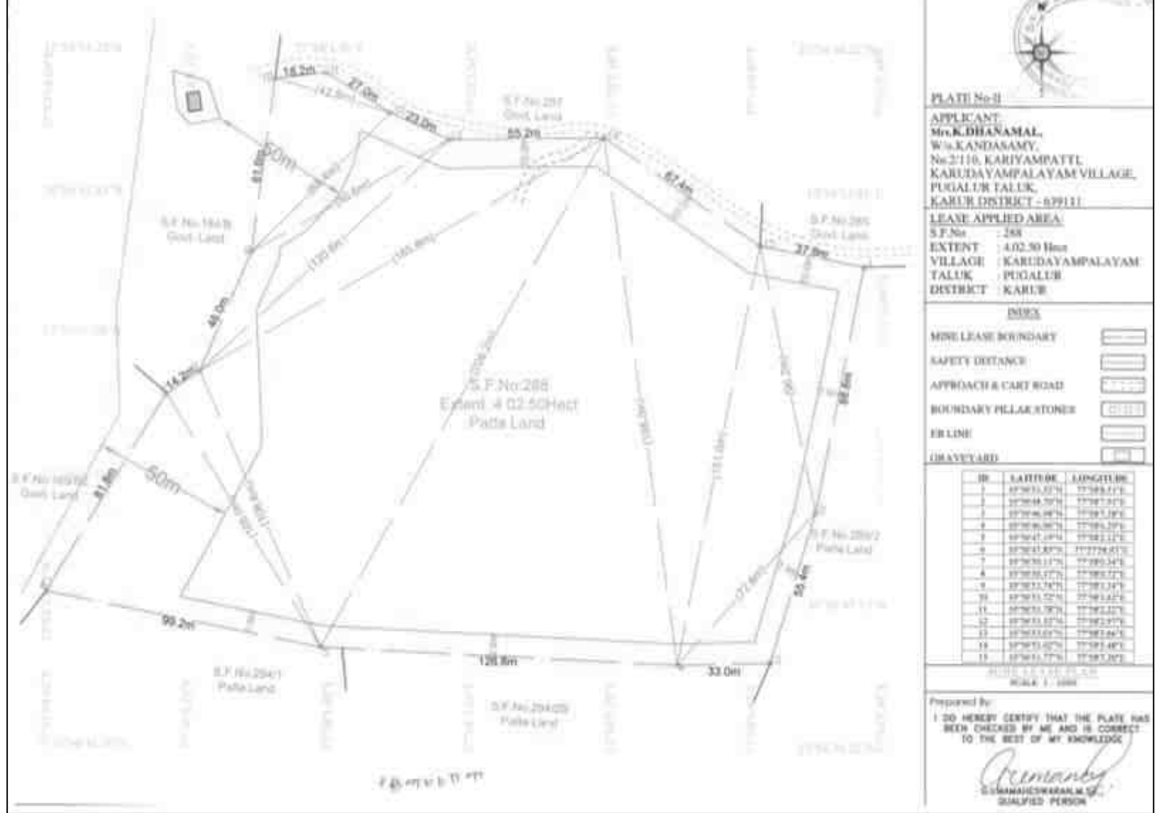
படம் 2.3 சுரங்க குத்தகை திட்டம்
