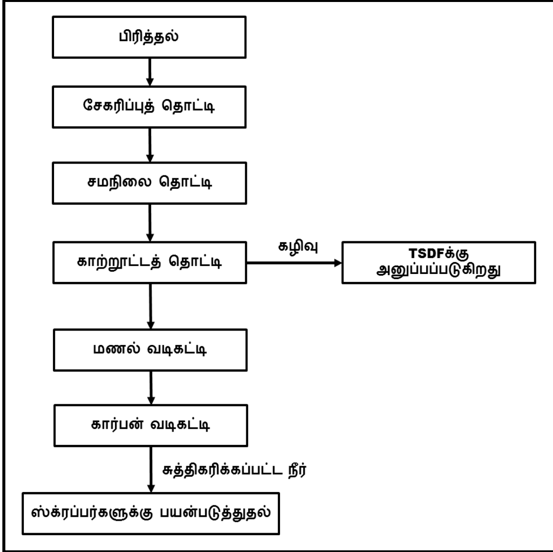
படம் 2.12 - கழிவுநீர் சுத்திகரிப்பு வசதி
