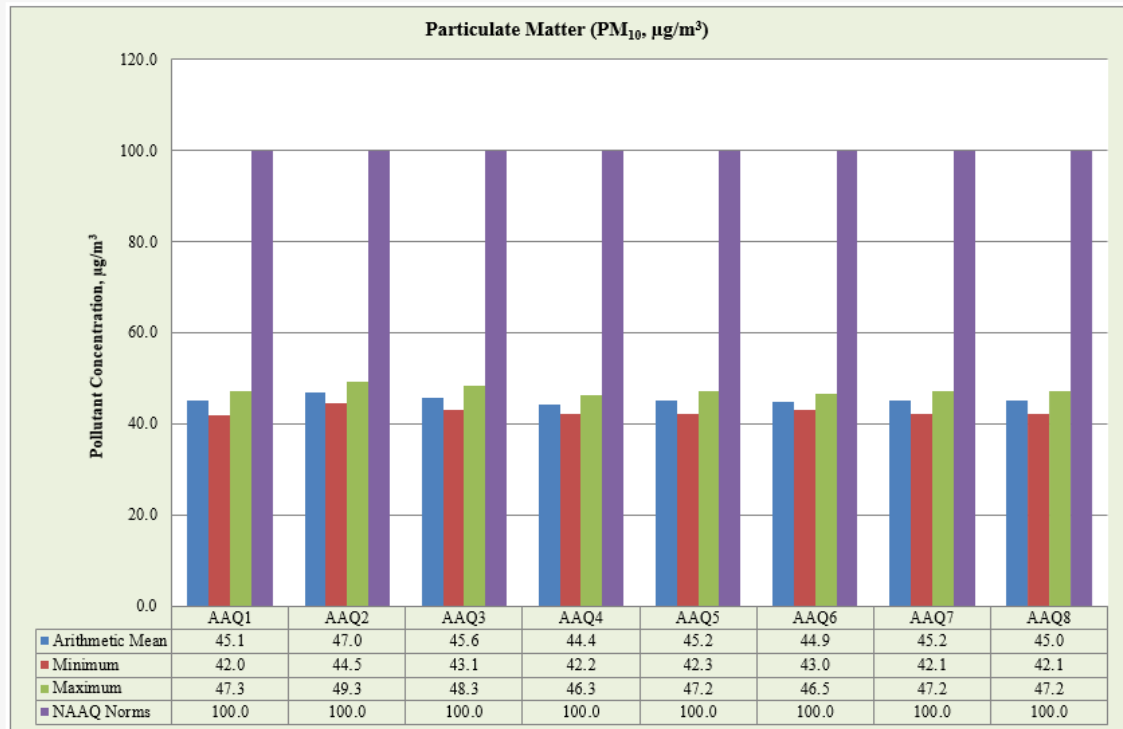
படம் 3.13 : பார்டிகுலேட் மேட்டரின் வரைபடம் (PM 10 )
