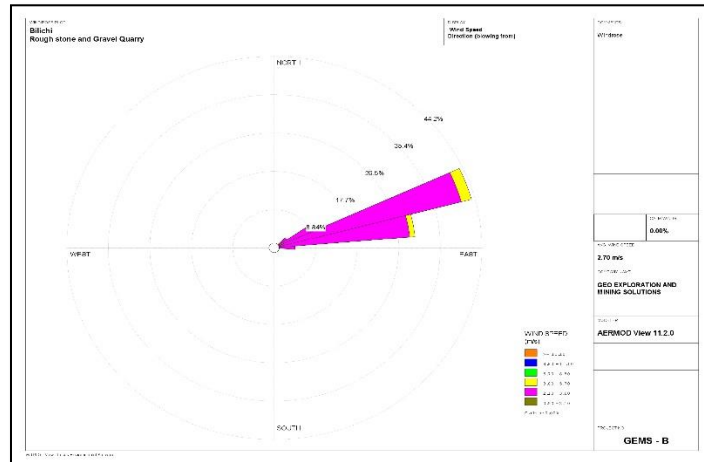
படம் 3.8: காற்று வீசும் திசையின் புகைப்படம்
